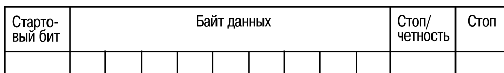
Рисунок 3.1 – Структура сообщения Modbus
