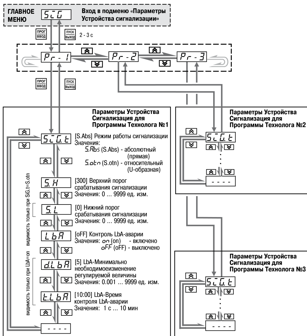
Рисунок 8.4 – Параметры устройства сигнализации
