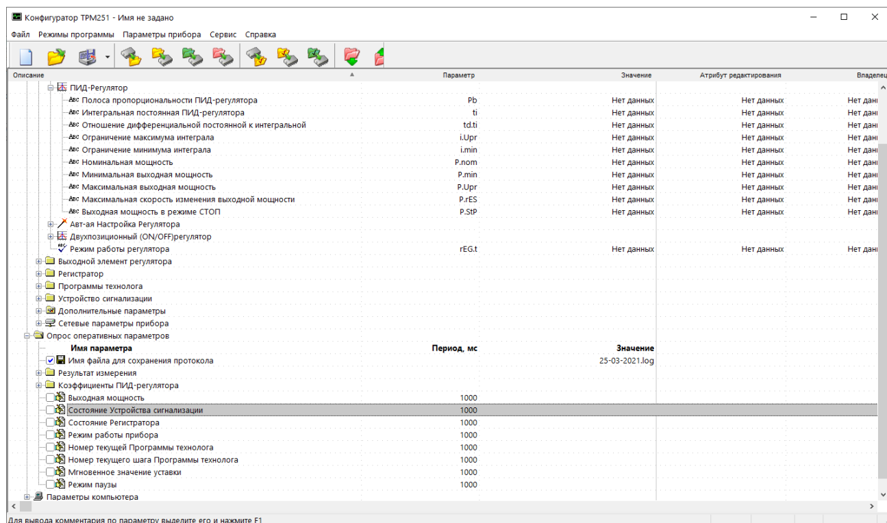
Рисунок 9.4 – Сохранение значений оперативных параметров в файл
