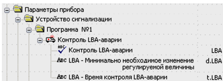
Рисунок 10.20 – Параметры t.LBA и d.LBA
