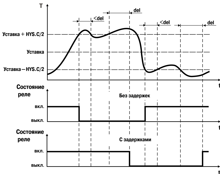
Рисунок 10.15 – Работа регулятора с заданными задержками
