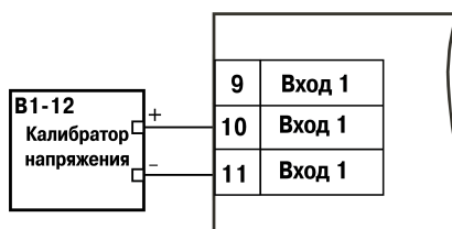
Рисунок 11.2 – Подключение калибратора напряжений
