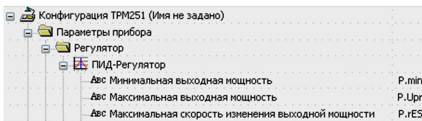
Рисунок 10.10 – Параметры настройки выходной мощности P.Upr, P.min и P.rES
