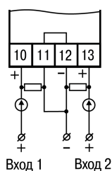
Рисунок 5.6 – Подключение активных датчиков
