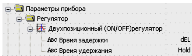
Рисунок 10.14 – Параметры Время задержки (dEL) и Время удержания (HoLd)
