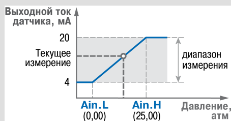
Рисунок 10.6 – Пример задания диапазона измерения
