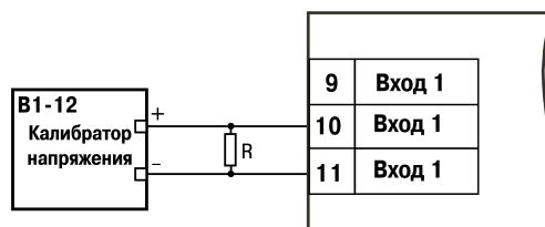
Рисунок 11.3 – Подключение калибратора напряжения 2
