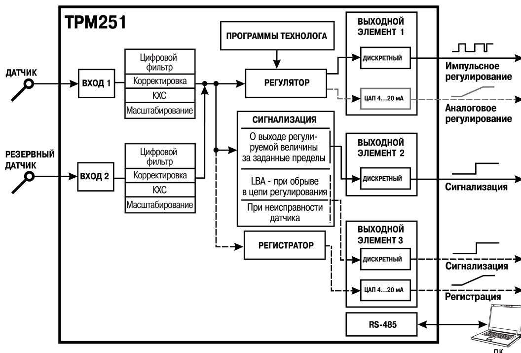
Рисунок 6.1 – Функциональная схема прибора
