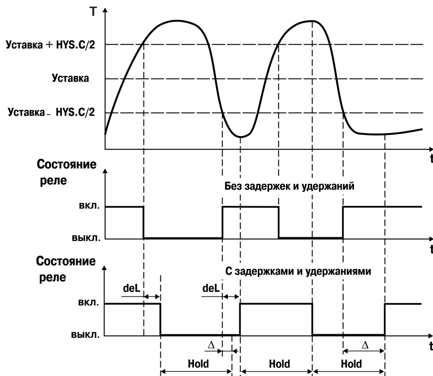
Рисунок 10.17 – Работа регулятора с заданным удержанием
