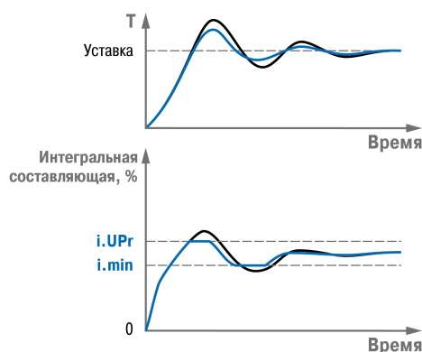
Рисунок 7.8 – Пример ПИД-регулирования
