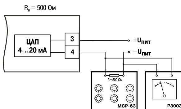
Рисунок 11.4 – Схема подключения к ВЭ типа «И»
