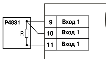
Рисунок 11.1 – Схема соединения с магазином сопротивлений
