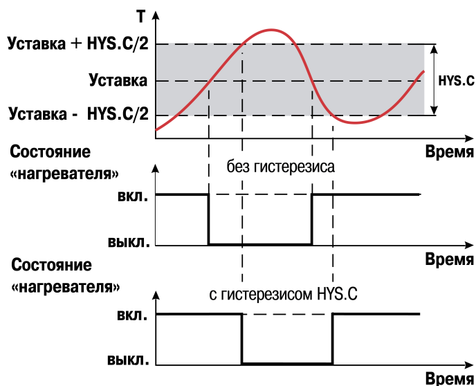
Рисунок 10.13 – Принцип работы двухпозиционного регулятора
