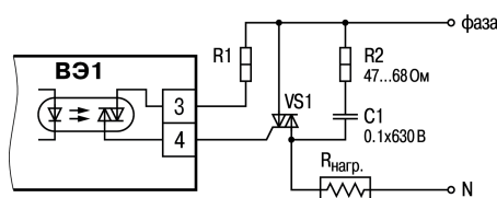
Рисунок 5.9 – Подключение к ВЭ нагрузки типа «С»
