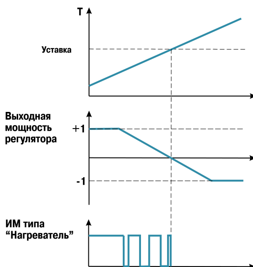
Рисунок 10.9 – Принцип формирования ШИМ-сигнала для «нагревателя»
