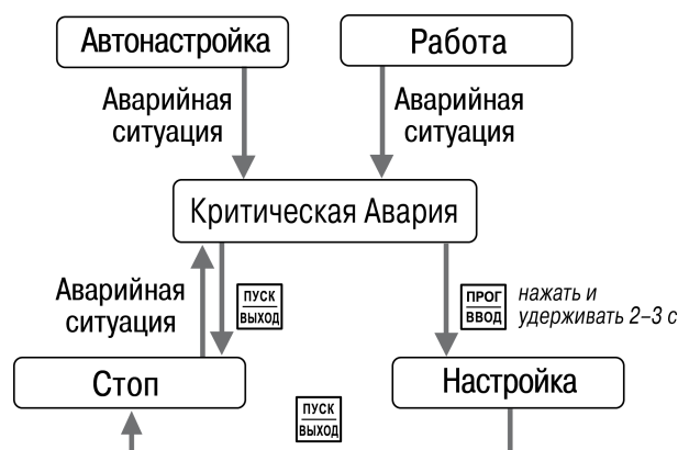
Рисунок 7.11 – Схема переключения режимов при Критической Аварии
