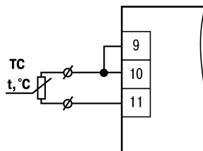
Рисунок 5.5 – Подключение ТС по двухпроводной схеме
