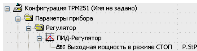
Рисунок 10.11 – Параметр выходная мощность в режиме Стоп (P.StP)
