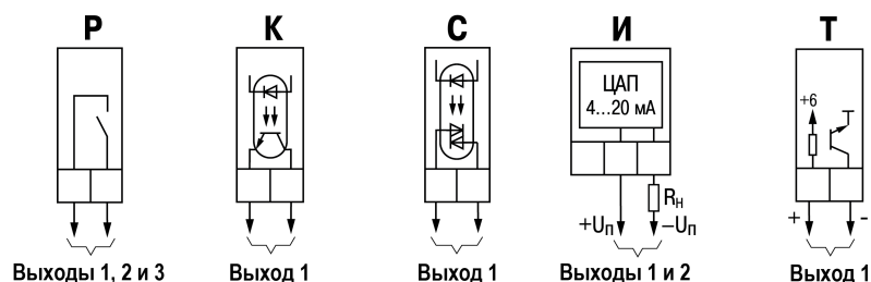
Рисунок 5.7 – Схема подключения к разным типам ВЭ
