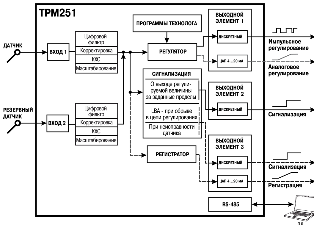
Рисунок 6.1 – Функциональная схема прибора
