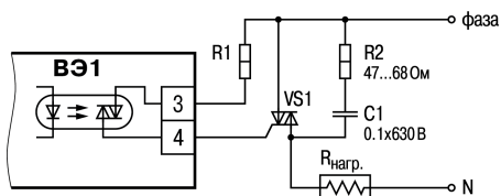
Рисунок 5.9 – Подключение к ВЭ нагрузки типа «С»
