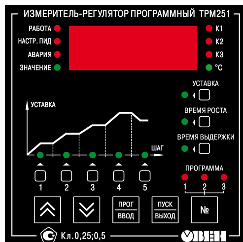
Рисунок 6.2 – Лицевая панель прибора
