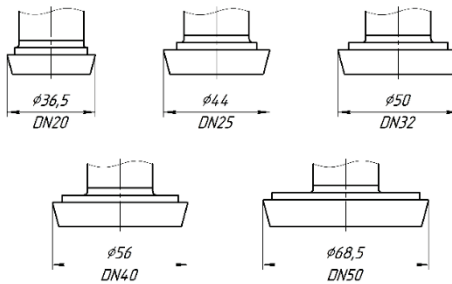
Рисунок А.2 – Габаритные и присоединительные размеры преобразователей ОВЕН ПД180-ДИ, -ДА, -ДВ, -ДИВ с присоединением молочная муфта DIN 11851
