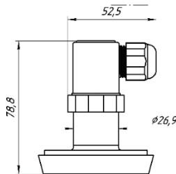
Рисунок А.1 – Габаритные и присоединительные размеры преобразователей ОВЕН ПД180-ДИ, -ДА, -ДВ, -ДИВ с присоединением Clamp DIN 32676
