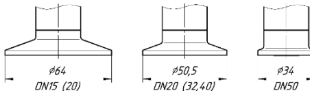
Рисунок А.1 – Габаритные и присоединительные размеры преобразователей ОВЕН ПД180-ДИ, -ДА, -ДВ, -ДИВ с присоединением Clamp DIN 32676
