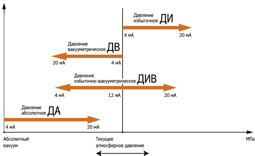
Рисунок 1.1 - Типы измеряемых давлений
