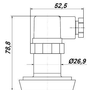
Рисунок 1 – Габаритные и присоединительные размеры ПД180-ДИ, -ДА, -ДВ, -ДИВ с присоединением Clamp DIN 32676
