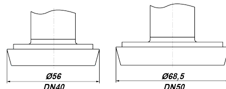
Рисунок 2 – Габаритные и присоединительные размеры ПД180-ДИ, -ДА, -ДВ, -ДИВ с присоединением молочная муфта DIN 11851
