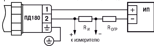
Рисунок 7 – Схема подключения
