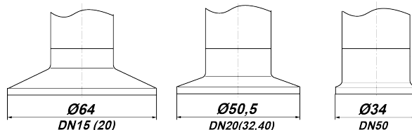
Рисунок 1 – Габаритные и присоединительные размеры ПД180-ДИ, -ДА, -ДВ, -ДИВ с присоединением Clamp DIN 32676
