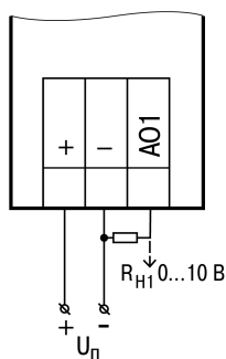
Рисунок 6.13 – Схема подключения к аналоговому выходу нагрузки в виде напряжения
