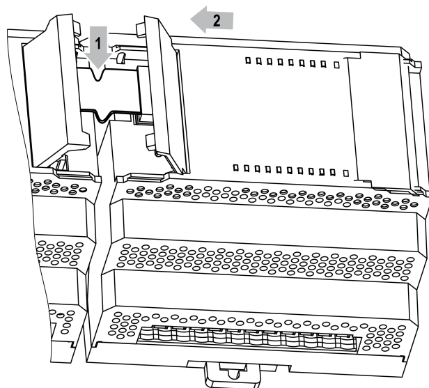
Рисунок 6.14 – Укладка шлейфа в углубление
