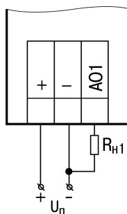
Рисунок 6.12 – Схема подключения к аналоговому выходу токовой нагрузки
