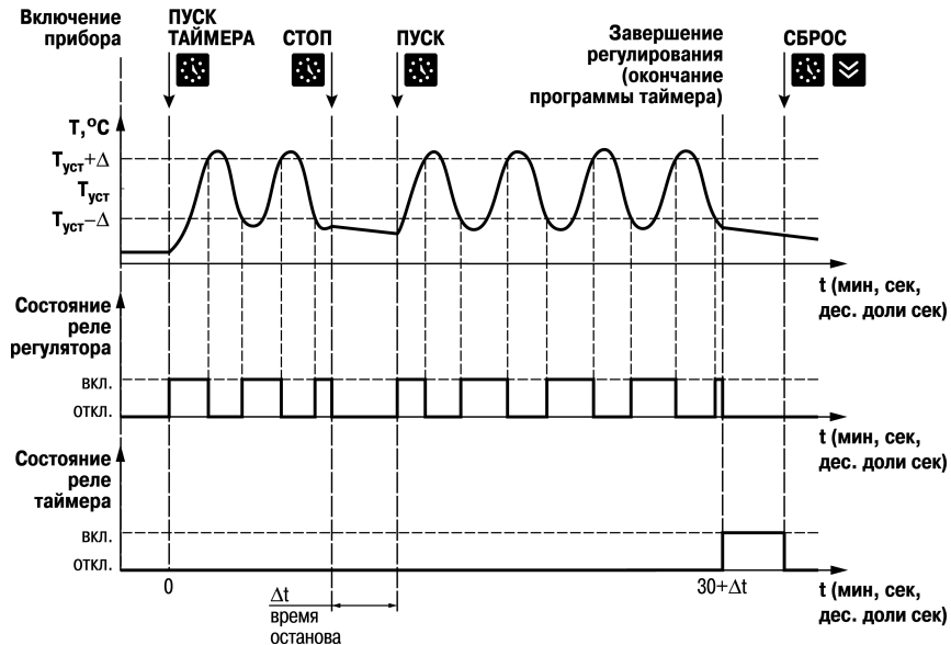
Рисунок 6.3 – График регулирования температуры по программе таймера
