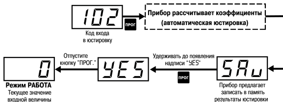
Рисунок 8.8 – Последовательность действий при юстировке схемы компенсации температуры свободных концов термопары
