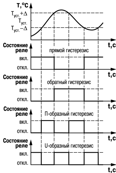
Рисунок 7.11 – Логика работы регулятора
