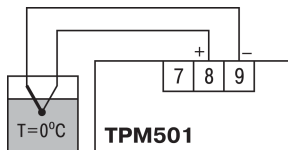
Рисунок 8.7 – Схема подключения
