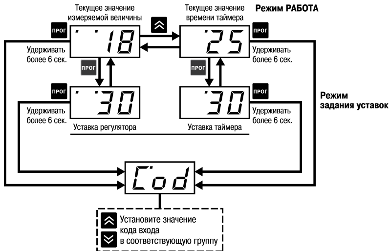
Рисунок 7.2 – Вход в режим установки параметров
