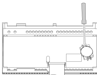
Рисунок 10.2 – Замена батарейки
