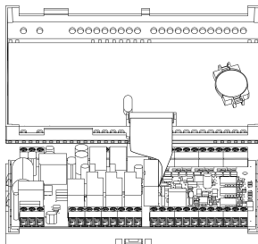
Рисунок 10.1 – Открытие корпуса
