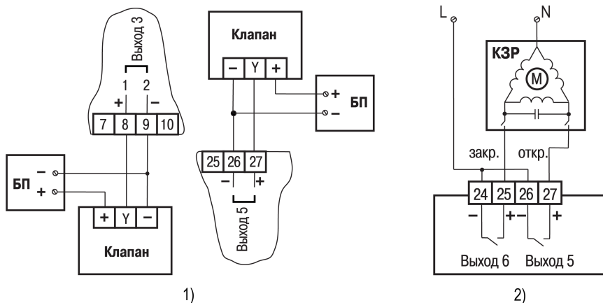
Рисунок 6.12 – Подключение клапана с аналоговым управлением к ВУ типа У (на примере подключения клапанов с приводами типа: 1) ST.0, 2) HR230-3)
