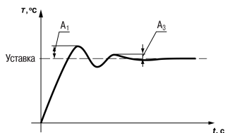
Рисунок Б.2 – График для определения ошибки регулирования
