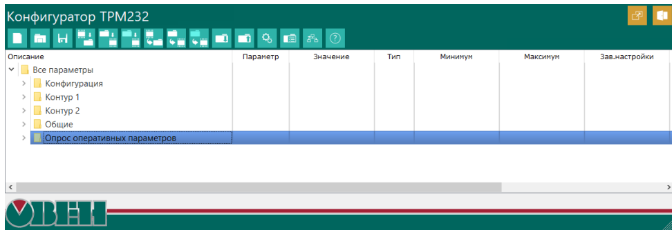
Рисунок 9.4 – Общий вид окна «Дерево параметров»
