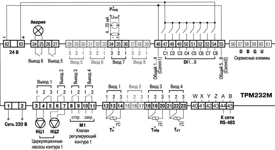
Рисунок 6.2 – Схема подключения для конфигурации № 2
