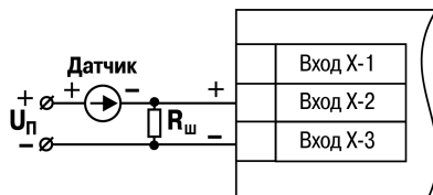
Рисунок 6.11 – Схема подключения пассивного датчика с токовым выходом 0...5 мА или 0 (4)...20 мА R_{ш} = 100 \pm 0,1 \text{ Ом}
