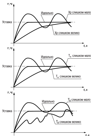
Рисунок Б.1 – Различные виды переходного процесса
