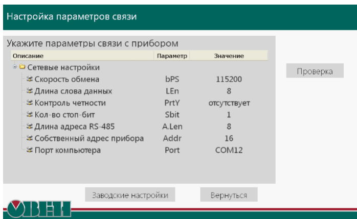
Рисунок 9.1 – Окно «Настройка параметров связи»
