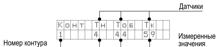
Рисунок 7.5 – Домашний экран контура
