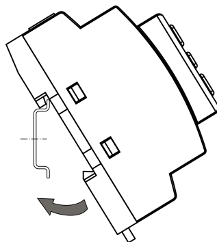
Рисунок 5.1 – Монтаж прибора на DIN-рейку
