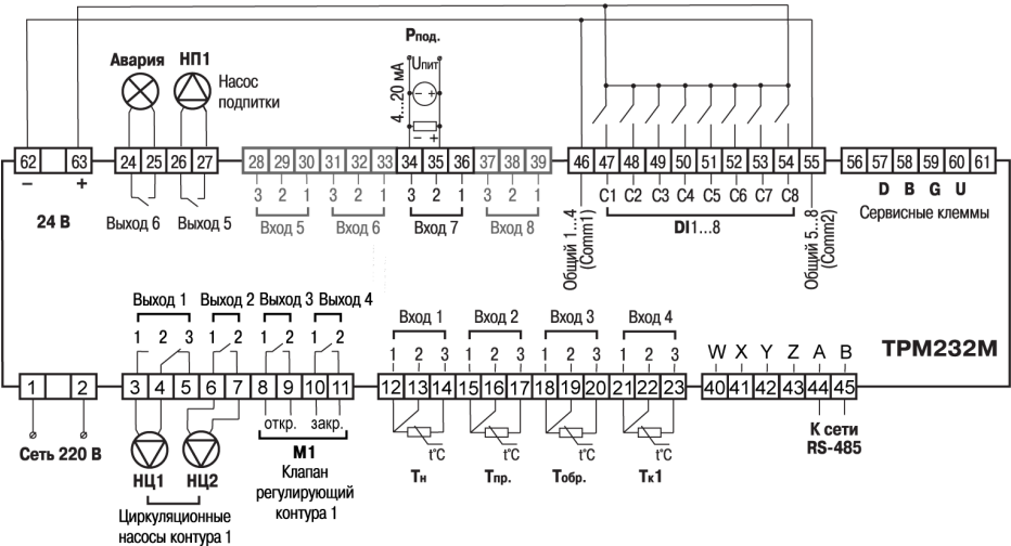
Рисунок 6.1 – Схема подключения для конфигурации № 1
