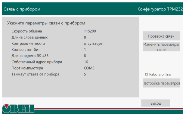
Рисунок 9.2 – Окно «Связь с прибором»
