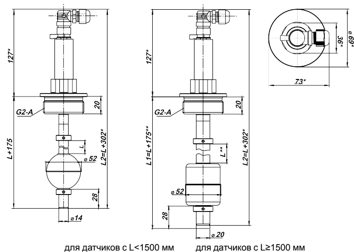
Рисунок 6.1 – Габаритные и присоединительные размеры
