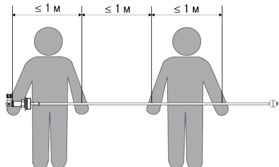
Рисунок 5.1 – Перемещение датчика длиной более 2 м
