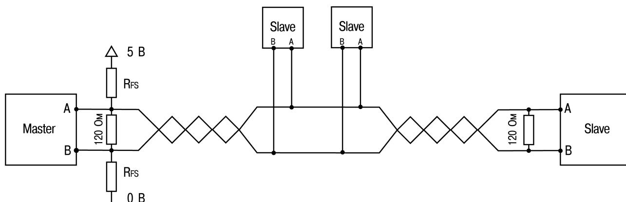
Рисунок 5.26 – Сеть RS-485 с подтягивающими резисторами
