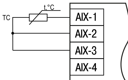
Рисунок 5.17 – Схема подключения ТС по трехпроводной схеме
