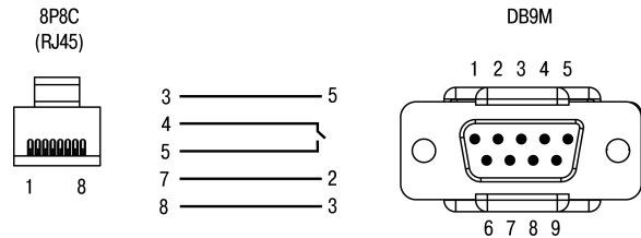
Рисунок 5.30 – Схема кабеля KC17
