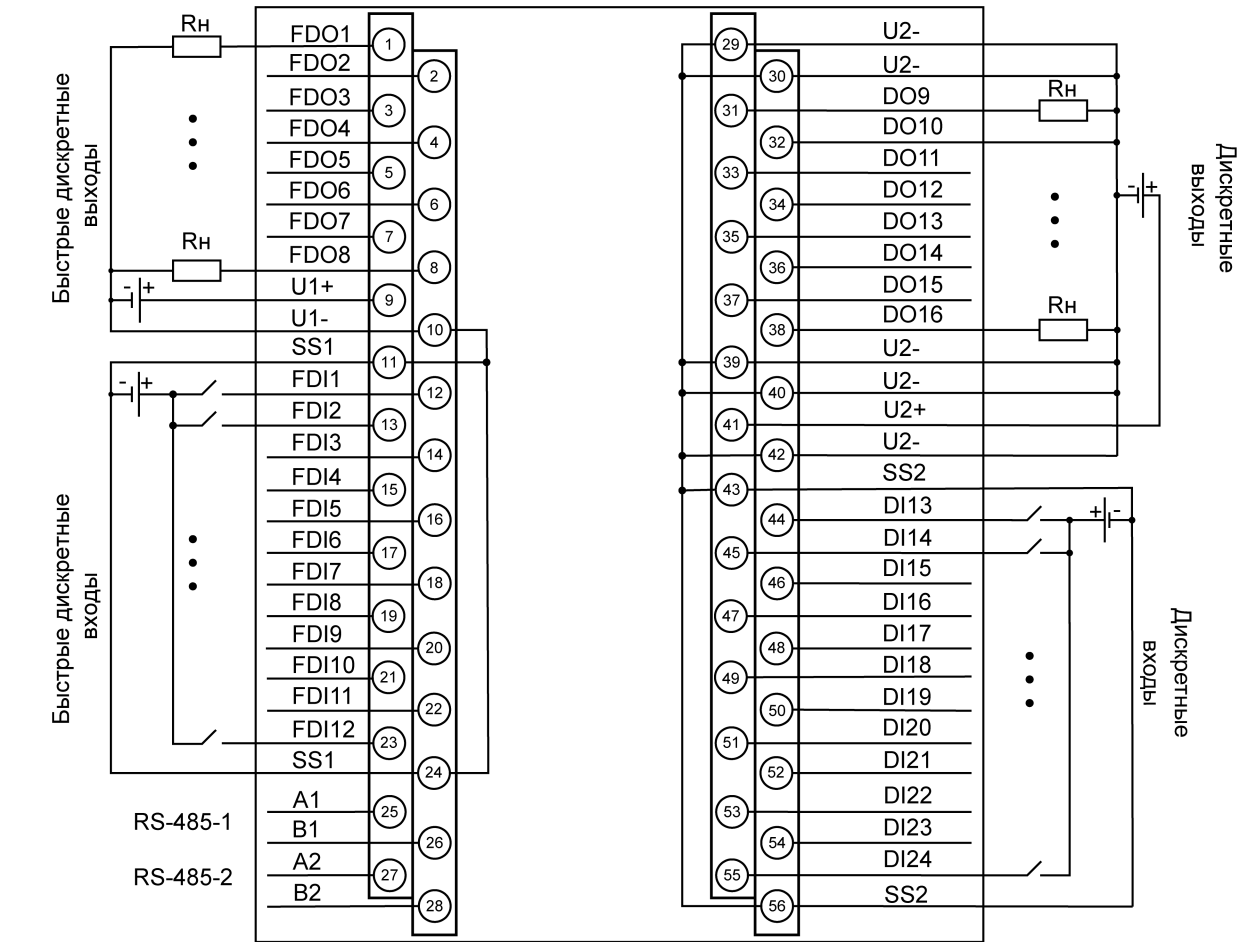
Рисунок 5.4 – Назначение контактов клеммника (модификация 03)
