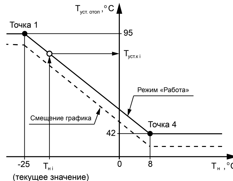
Рисунок 10.3 – Отопительный график
