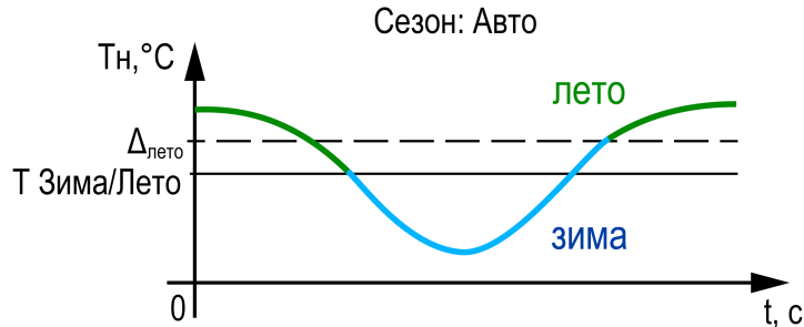
Рисунок 10.11 – Определение сезона
