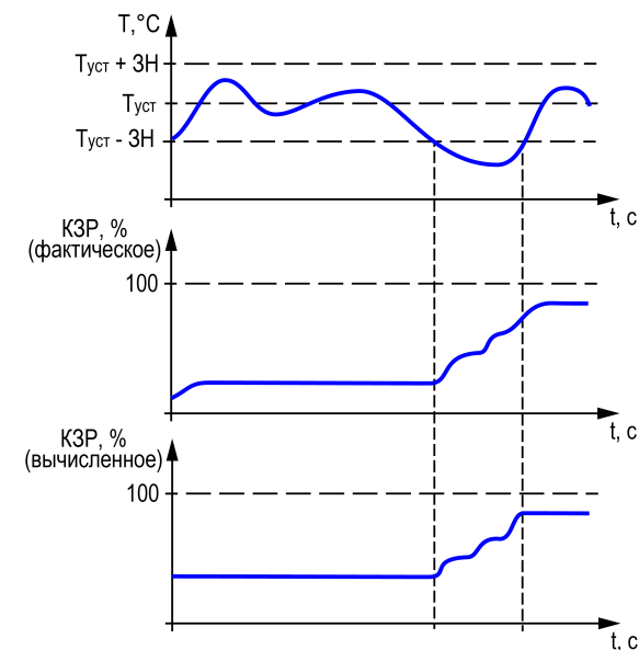
Рисунок 10.1 – Принцип работы КЗР
