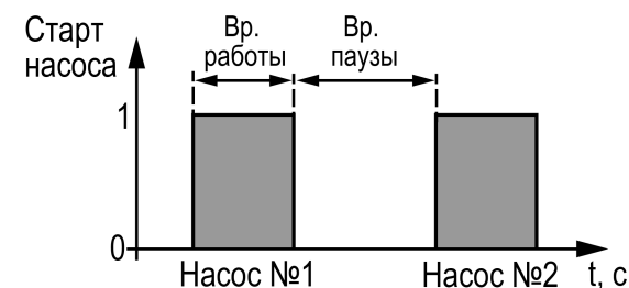
Рисунок 10.9 – Чередование насосов
