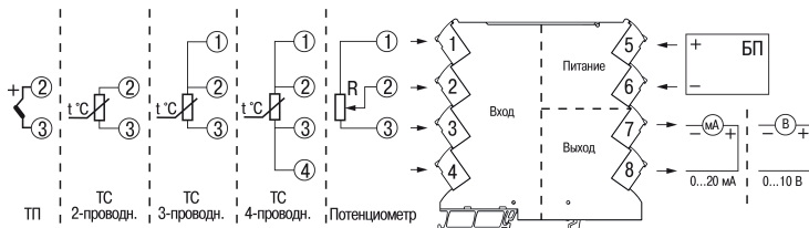
Рисунок 6.3 – Подключение прибора
