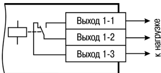
Рисунок Б.15 – Схема подключения нагрузки к ВЭ типа «Р» (для первого ВЭ)
