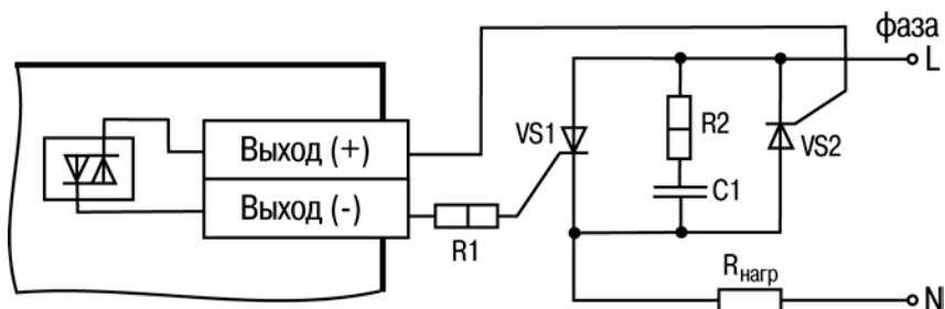
Рисунок Б.13 – Схема подключения нагрузки к ВЭ типа «С» двух тиристоров, подключенных встречно-параллельно (R2=47... 68 Ом, C1=0.1мкфx630 В)
