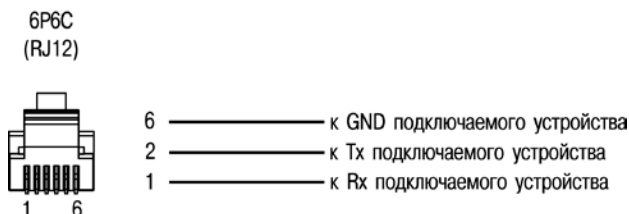
Рисунок В.3 – Схема кабеля для подключения ПЛК63 к порту RS-232
