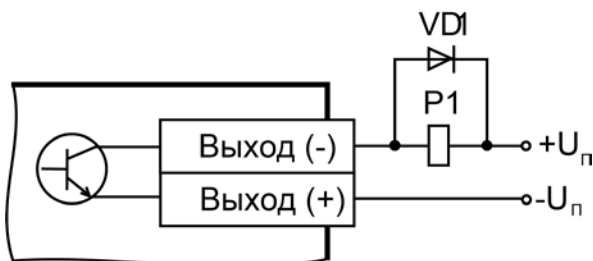
Рисунок Б.11 – Схема подключения нагрузки к ВЭ типа «К» (диод VD1 должен быть рассчитан на напряжение 100 \text{ В} и ток 1 \text{ А} )
