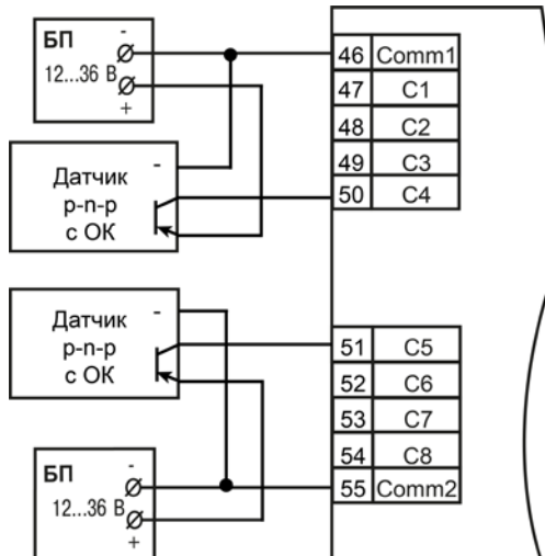
Рисунок Б.2 – Схема подключения р-н-р датчиков
