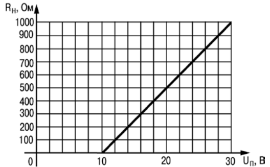
Рисунок 3.4 – График зависимости R_n(U_p)
