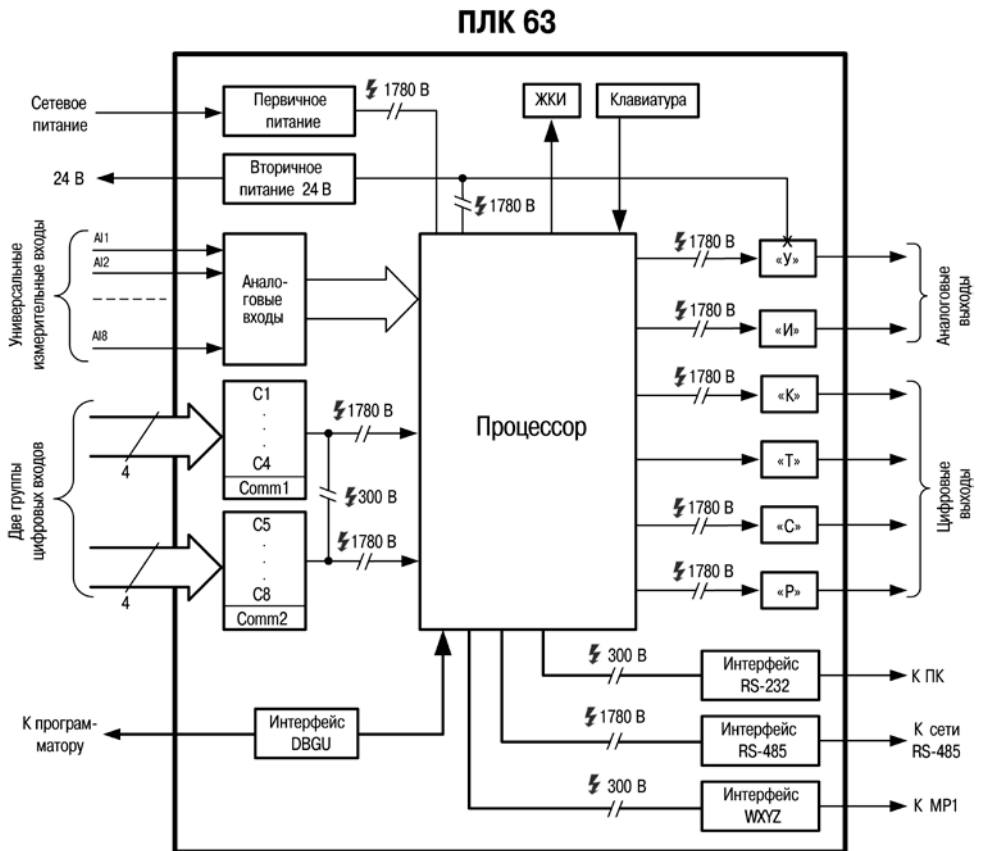
Рисунок 3.2 – Функциональная схема прибора
