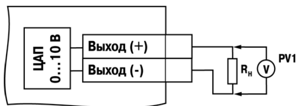
Рисунок Б.8 – Схема подключения нагрузки к ВЭ типа «У». R_{\text{н}} > 2 \text{ кОм}
