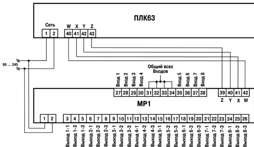
Рисунок Б.16 – Схема подключения модуля МР1 к ПЛК63
