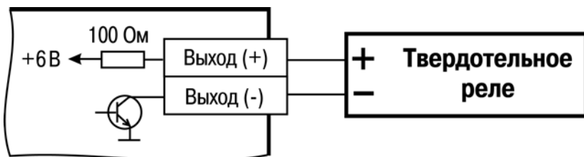
Рисунок Б.14 – Схема подключения нагрузки к ВЭ типа «Т»
