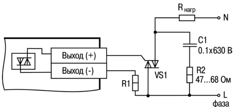
Рисунок Б.12 – Схема подключения нагрузки к ВЭ типа «С»
