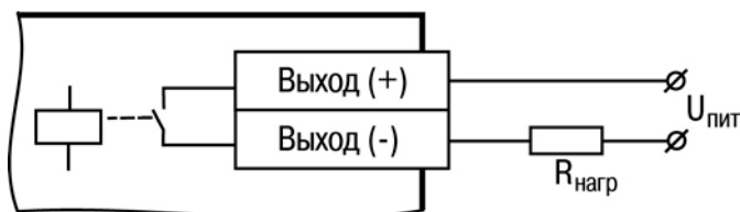
Рисунок Б.10 – Схема подключения нагрузки к ВЭ типа «Р»
