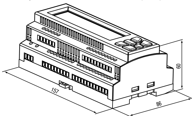
Рисунок 5.2 – Габаритные размеры корпуса
