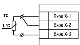
Рисунок 6.7 – Трехпроводная схема подключения ТС
