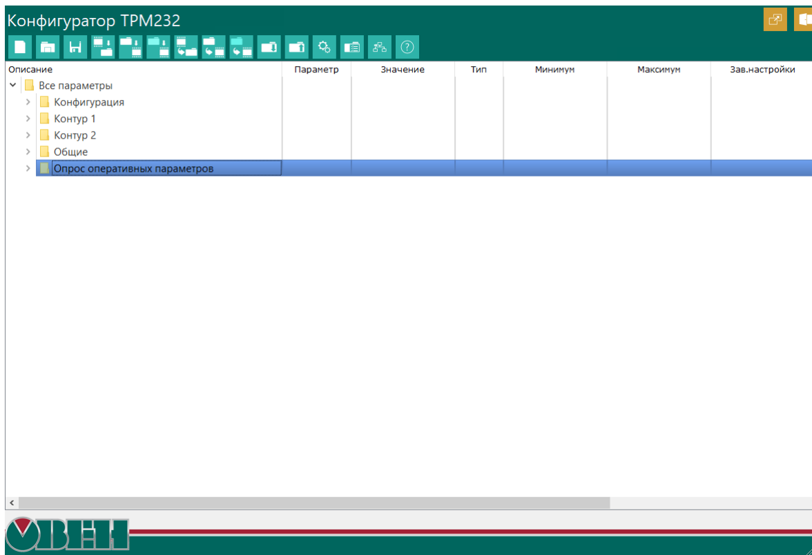
Рисунок 9.4 – Общий вид окна «Дерево параметров»
