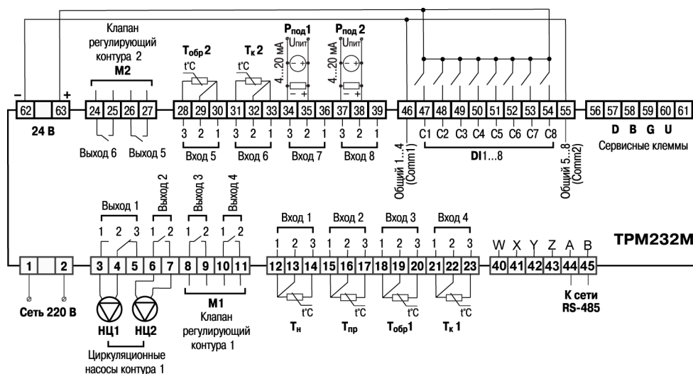
Рисунок 6.3 – Схема подключения для конфигурации № 3
