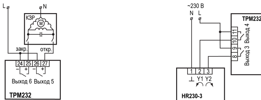
Рисунок 6.13 – Подключение клапана с дискретным управлением к ВУ типа Р
