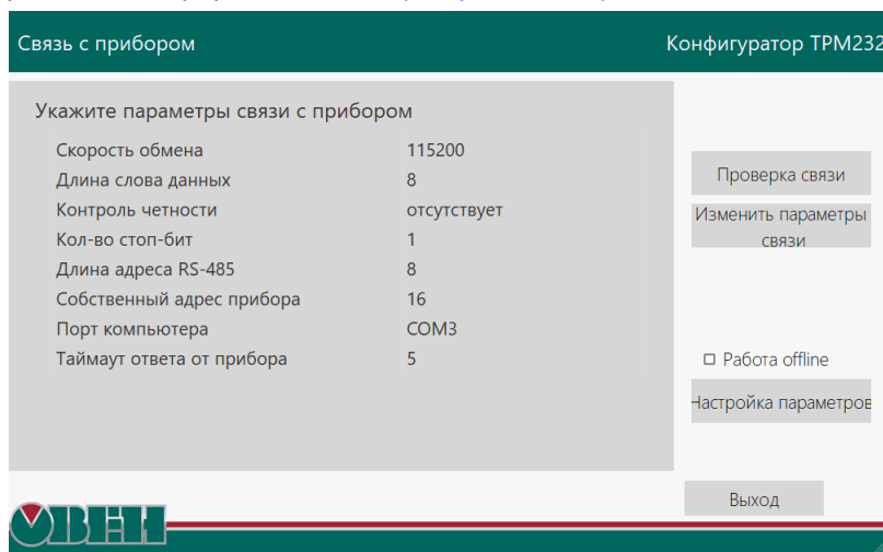
Рисунок 9.2 – Окно «Связь с прибором»
