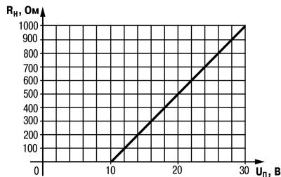
Рисунок 5.16 – График зависимости R_H ( U_n )
