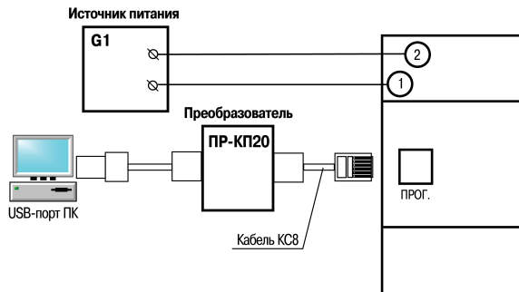
Рисунок 5.18 – Схема подключения к ПК (через преобразователь ПР-КП20), G1 – источник питания с номинальным напряжением, зависящим от исполнения прибора
