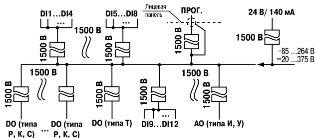
Рисунок 5.3 – Схема прочности гальванической изоляции входов/выходов
