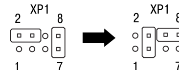
Рисунок 4.4 – Изменение конфигурации перемычек
