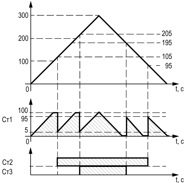
Рисунок 7.7 – Управление электрическим нагревателем
