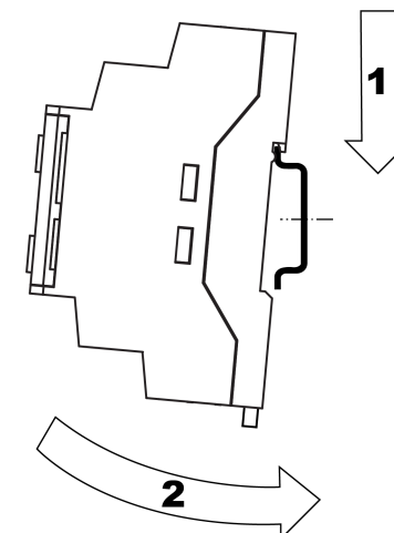
Рисунок 10.1 – Монтаж и демонтаж прибора
