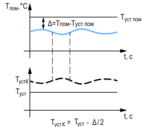
Рисунок 7.12 – Каскадное регулирование
