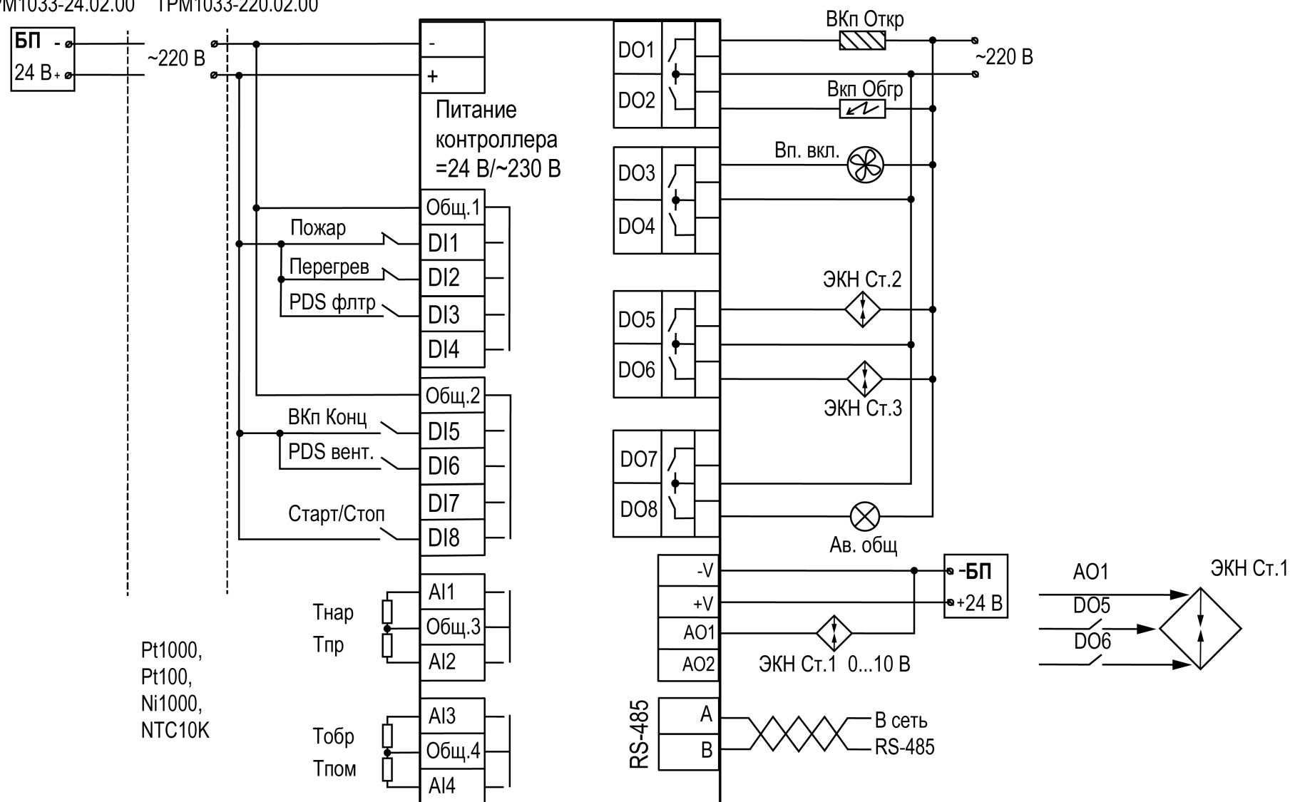
Рисунок 13.2 – Схема подключения Алгоритм 02.00 (Система с электрическим калорифером нагрева)
