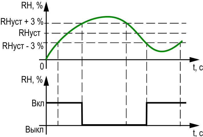
Рисунок 7.9 – Управление увлажнителем
