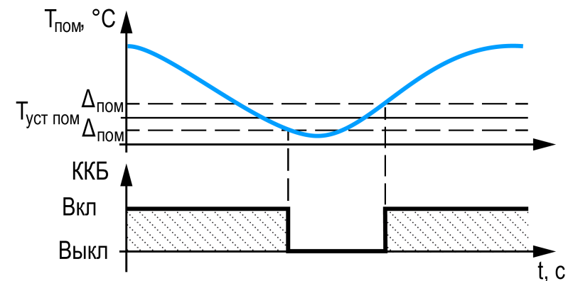
Рисунок 7.10 – Управление ККБ
