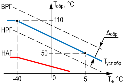
Рисунок 7.4 – График Тобр(Тн)
