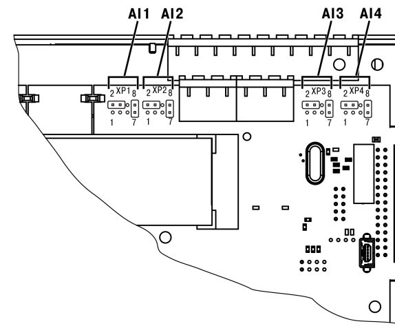
Рисунок 4.3 – Расположение входов
