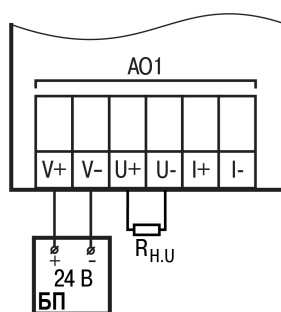
Рисунок 5.12 – Схема подключения к АО ПРМ-х.3 типа У
