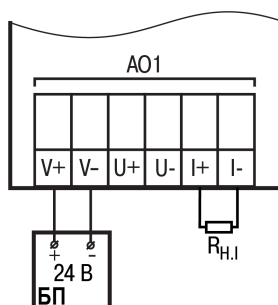
Рисунок 5.11 – Схема подключения к АО ПРМ-х.3 типа И (0(4)...20 мА)
