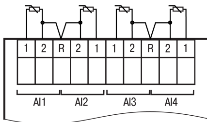
Рисунок 5.6 – Подключение ТС к аналоговым входам (AI) ПРМ-х.3
