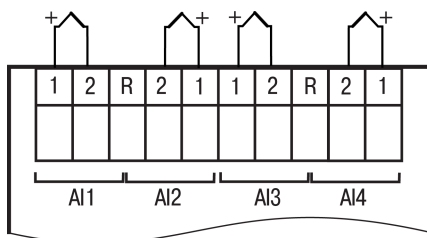
Рисунок 5.7 – Подключение ТП к AI ПРМ-х.3
