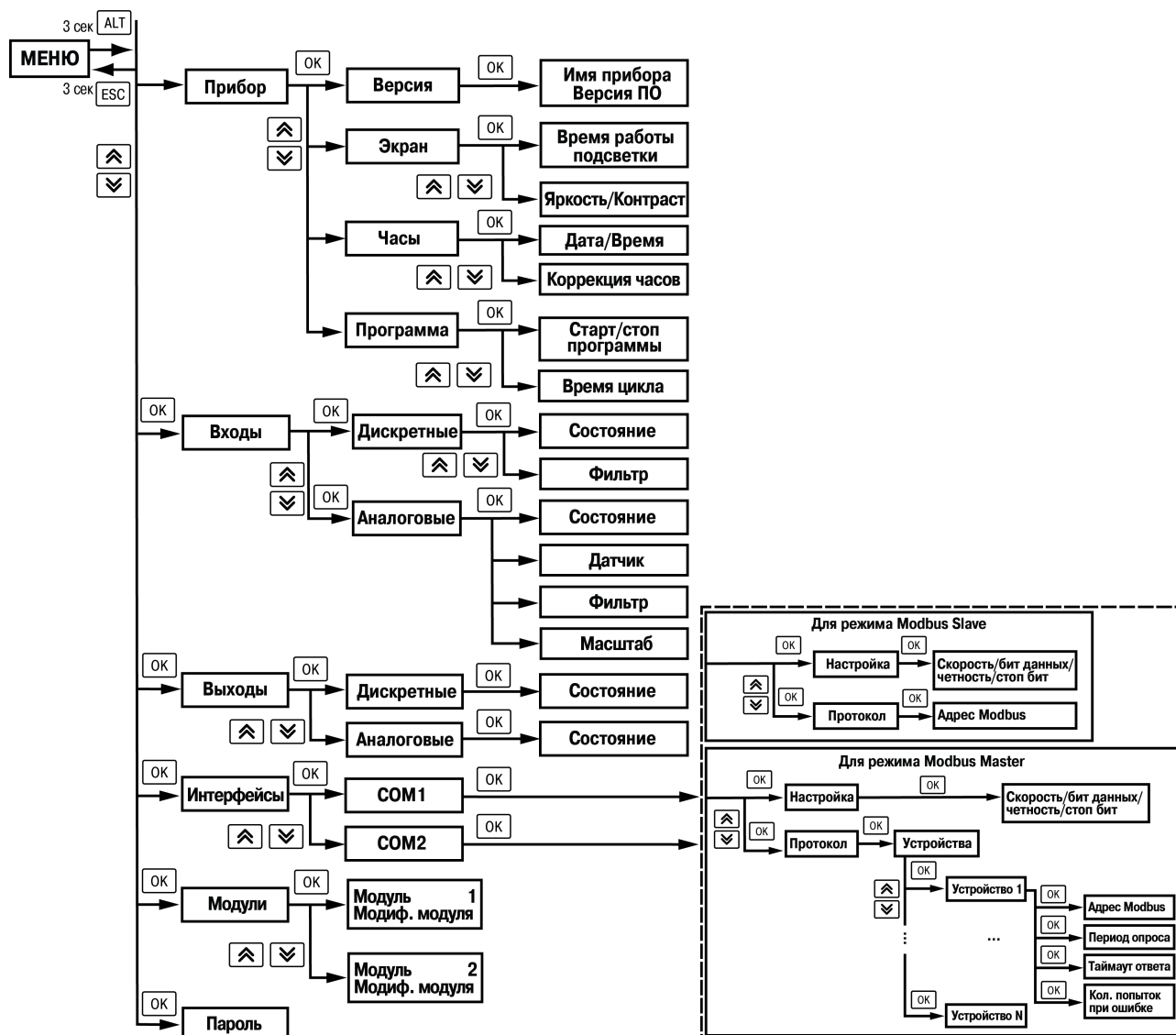
Рисунок 7.2 – Структура системного меню
