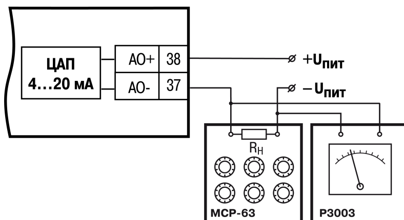
Рисунок 8.10 – Схема подключения к ВЭ типа «И» (R н = 500 Ом)
