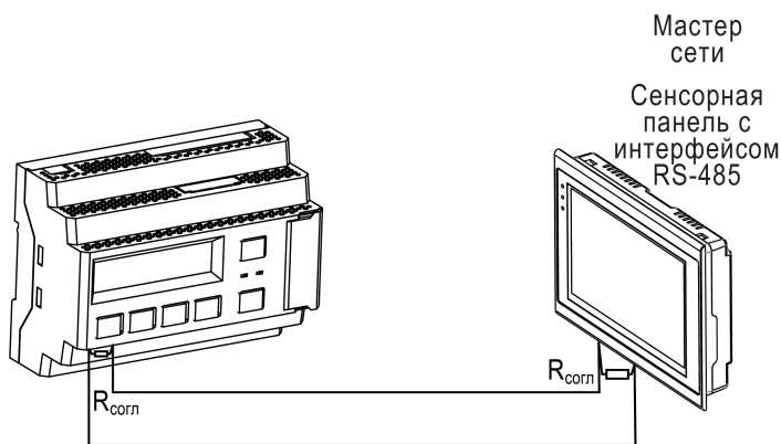
Рисунок 5.16 – Типовая схема подключения для PR200 в режиме Slave
