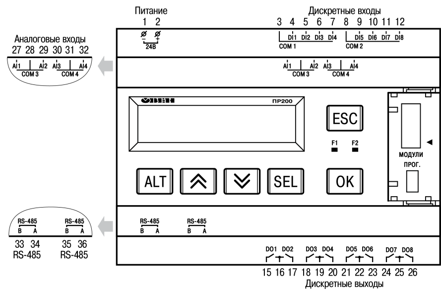
Рисунок А.13 – Расположение контактов ПР200-24.3.2.X
