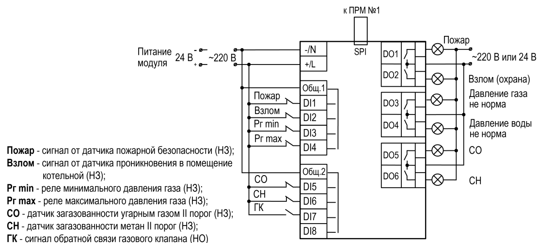
Рисунок 6.6 – Схема подключения к ПРМ-х.1 сигналов общекотельных аварий
