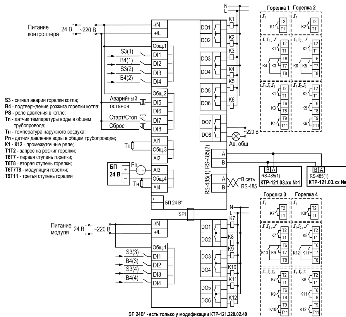
Рисунок 6.4 – Схема подключения КТР-121.02.40 и ПРМ-х.1 для управления котельной с четырьмя котлами и ГВС
