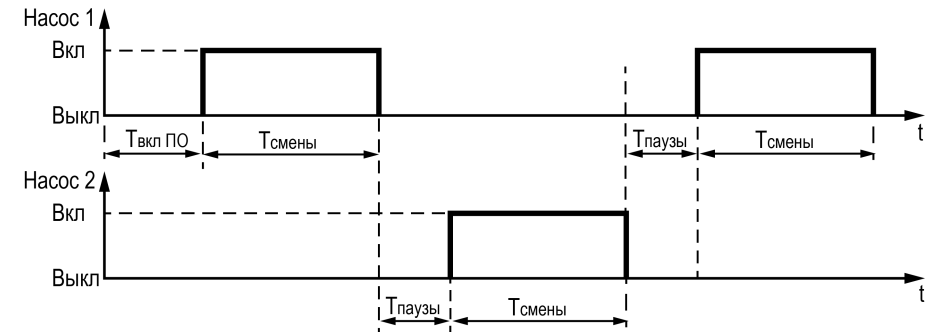
Рисунок 8.1 – Чередование насосов
