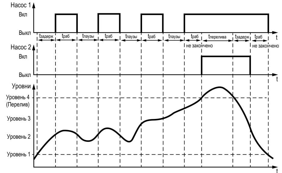
Рисунок 8.5 – Авария дискретных датчиков уровня
