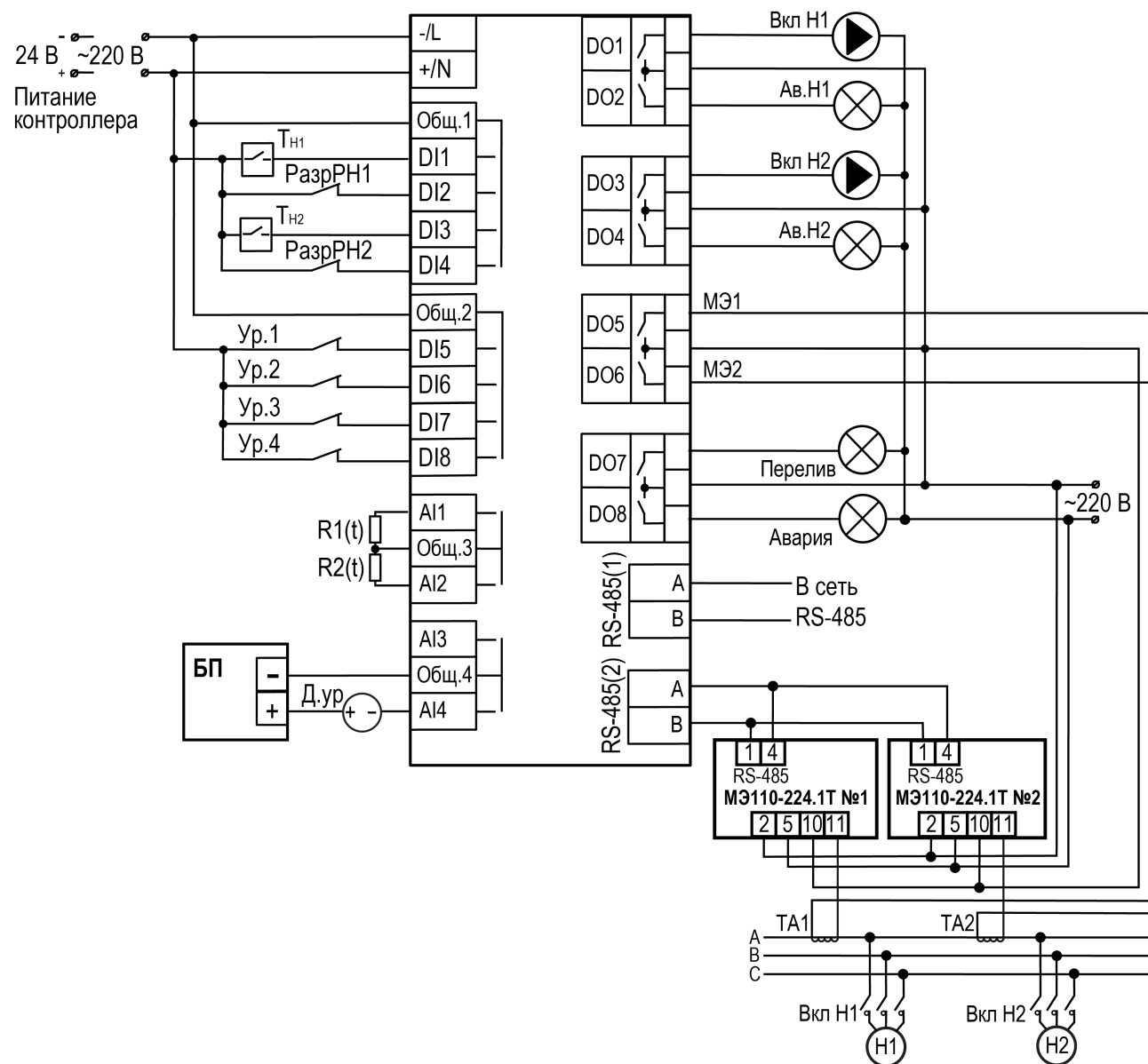
Рисунок 4.4 – Схема подключения СУНА-121.X.09.00
