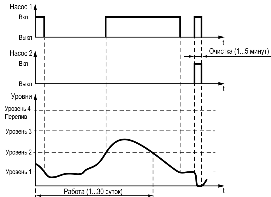
Рисунок 8.3 – Очистка от стоков
