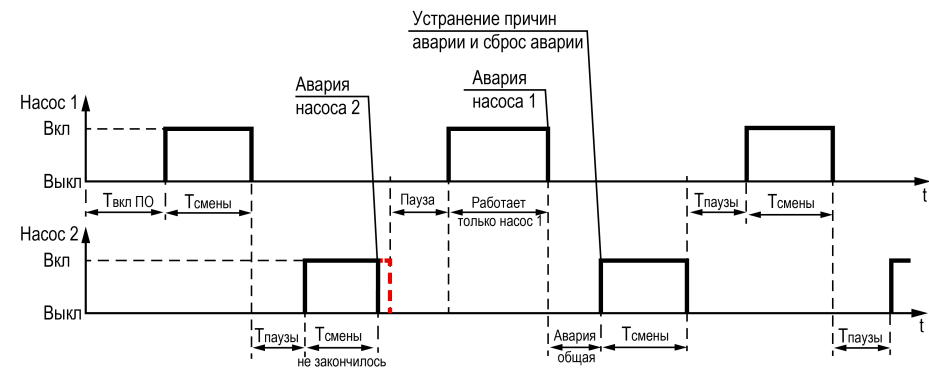
Рисунок 8.4 – Авария насосов
