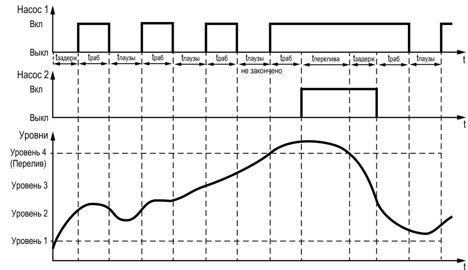
Рисунок 8.6 – Авария аналогового датчика уровня
