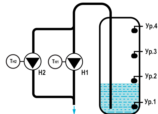
Рисунок 1.1 – Схема объекта управления
