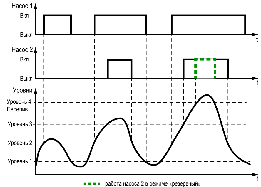
Рисунок 8.2 – Регулирование уровня
