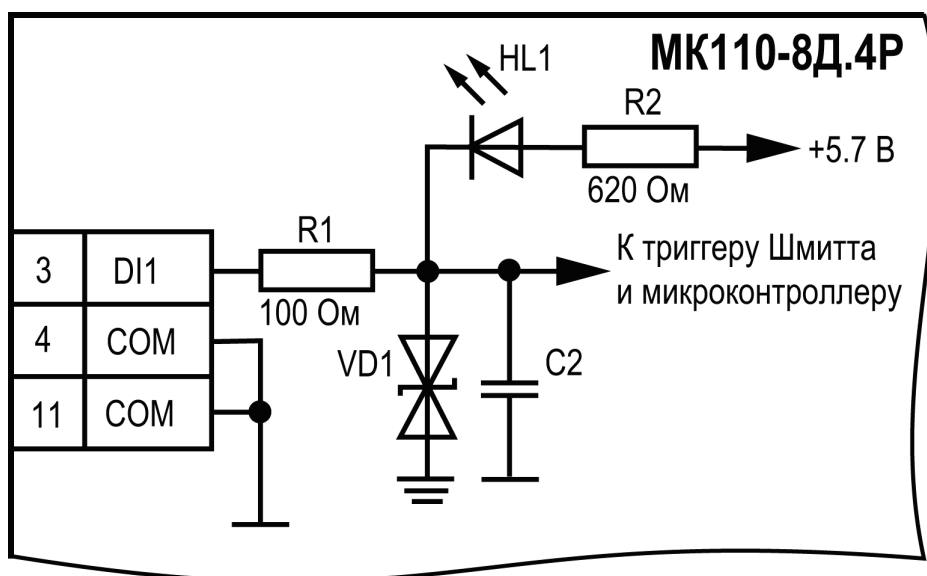
Рисунок 5.9 – Электрическая принципиальная схема группы дискретных входов МК110-224.8Д.4Р (схема других групп входов идентична приведенной)
