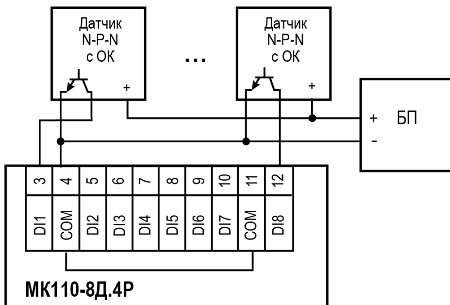
Рисунок 5.5 – Схема подключения трехпроводных дискретных датчиков, имеющих выходной транзистор n-p-n типа с открытым коллектором
