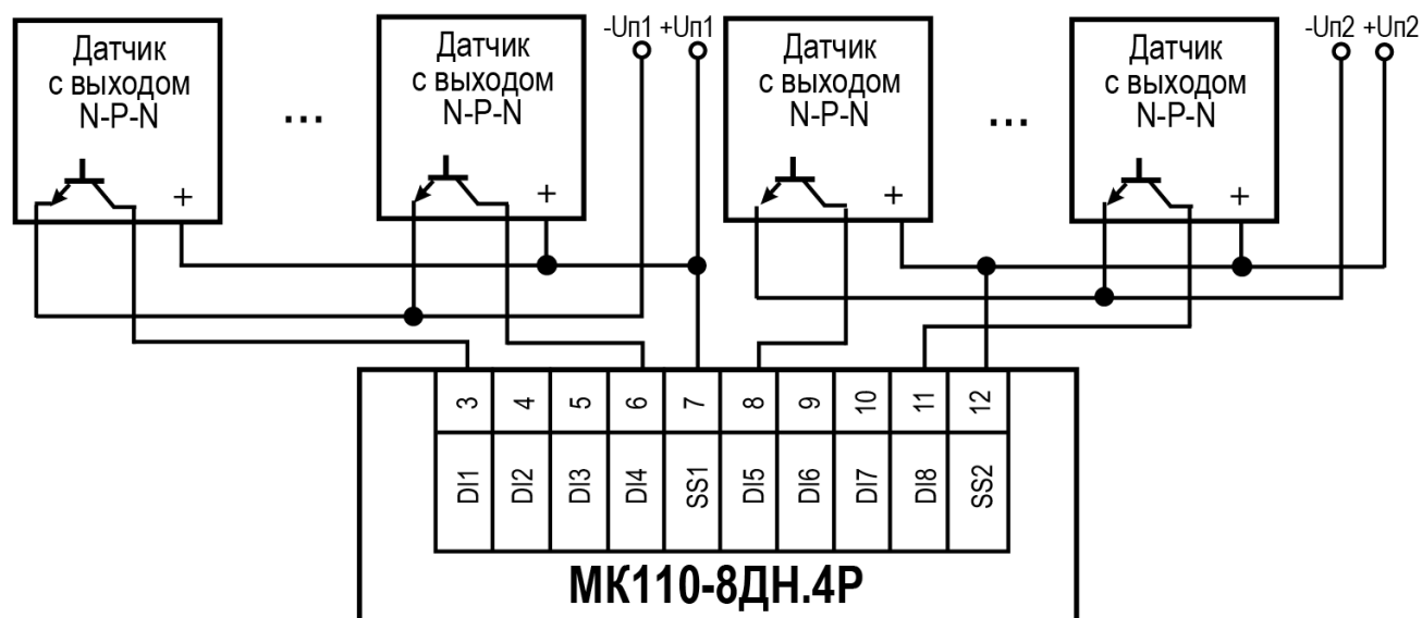
Рисунок 5.7 – Схема подключения дискретных датчиков с транзисторным выходом n-p-n типа с открытым коллектором
