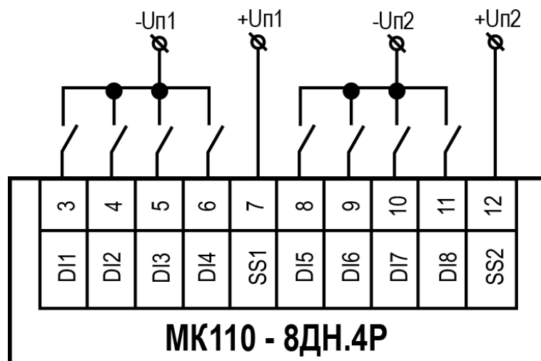
Рисунок 5.6 – Схема подключения дискретных датчиков с выходом типа «сухой контакт»
