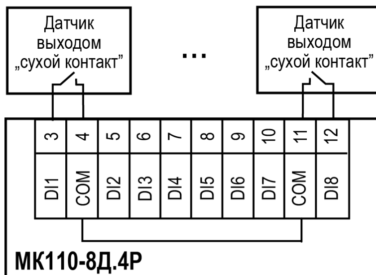
Рисунок 5.4 – Схема подключения дискретных датчиков с выходом типа «сухой контакт»
