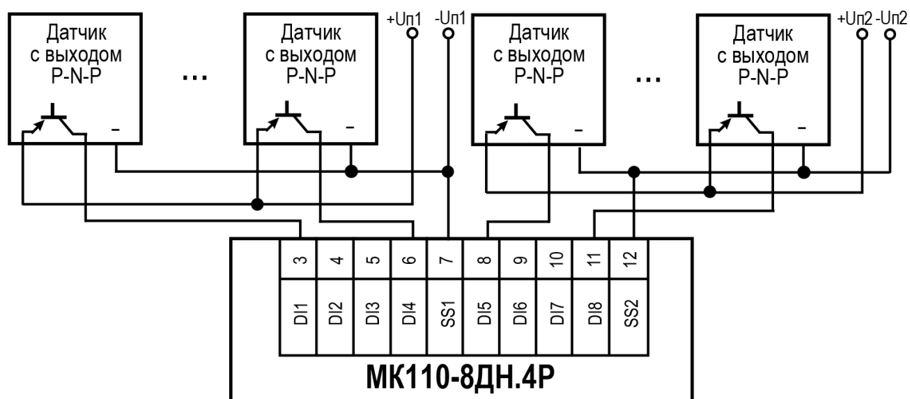
Рисунок 5.8 – Схема подключения дискретных датчиков с транзисторным выходом p-n-p типа
