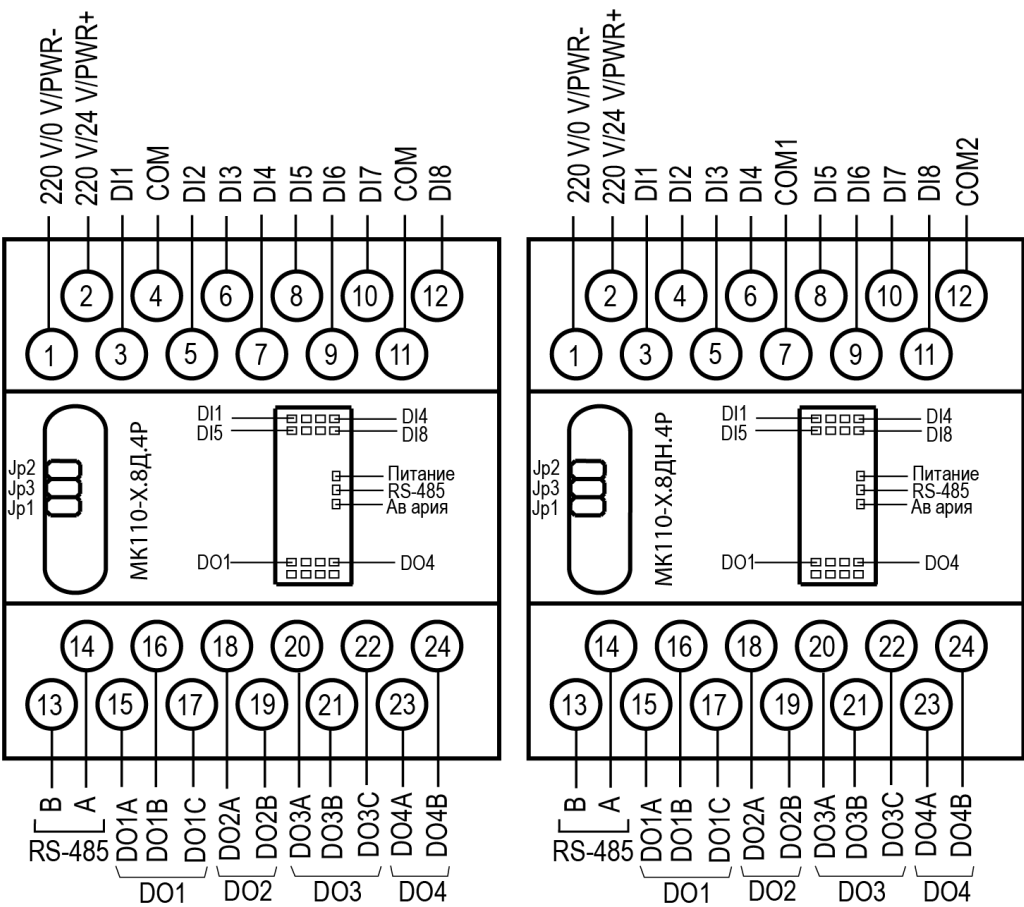
Рисунок 5.2 – Назначение контактов клеммника
