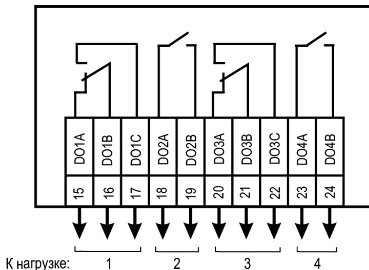
Рисунок 5.3 – Схема подключения ВЭ типа электромагнитное реле
