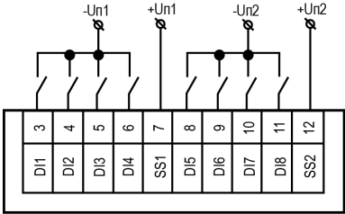
Рисунок 2 – Подключение датчиков с выходом типа «сухой контакт»
