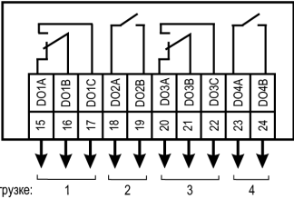
Рисунок 5 – Подключение к выходам типа электромагнитное реле
