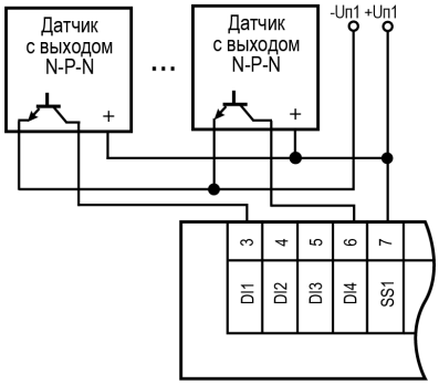
Рисунок 3 – Подключение датчиков с выходным транзистором п-п-п типа с открытым коллектором
