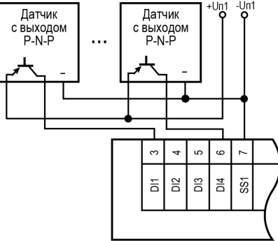
Рисунок 4 – Подключение датчиков с выходным транзистором р-п-п типа
