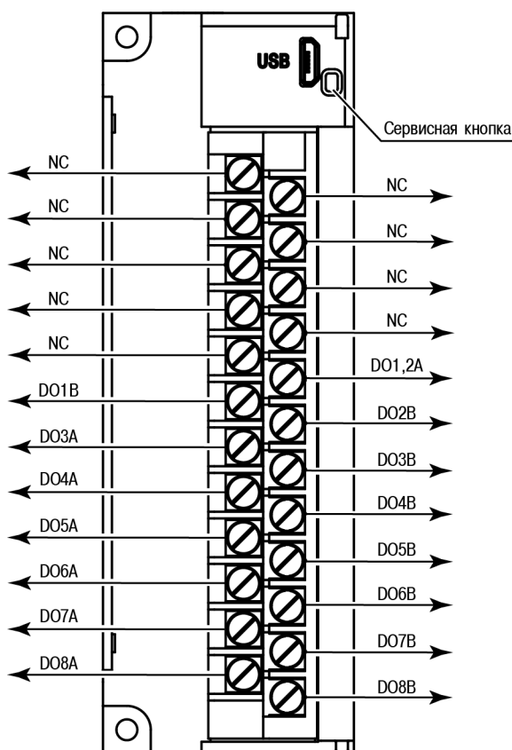
Рисунок 5.1 – Назначение контактов клеммника
