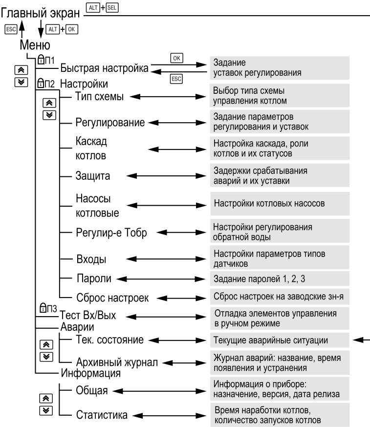
Рисунок 9.1 – Схема переходов по меню
