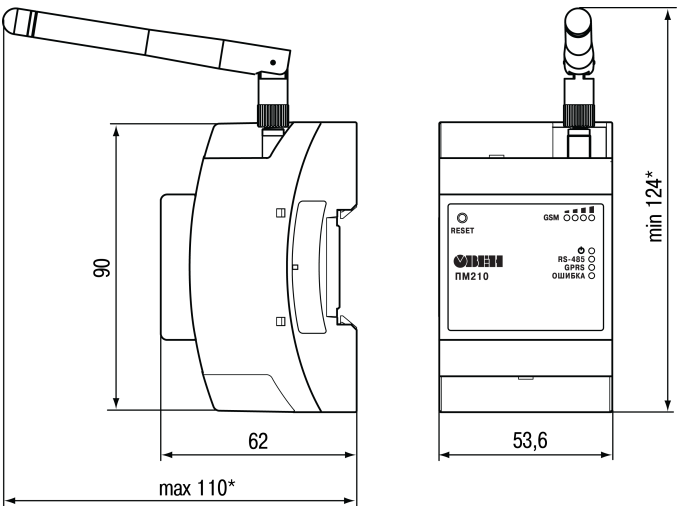
Рисунок 4 – Габаритные размеры ПМ210
