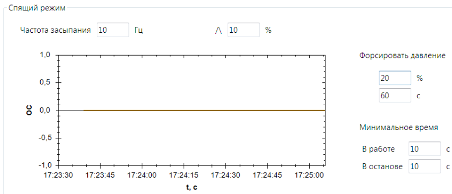
Рисунок 6.11 - Окно настройки «Спящего» режима ПЧВЗ
