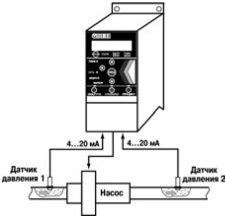
Рисунок 4.6 - Схема установки
