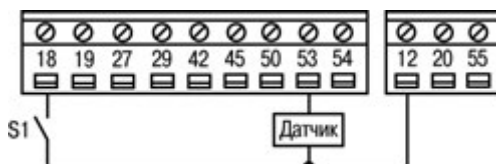
Рисунок 4.8 - Схема внешних подключений ПЧВЗ
