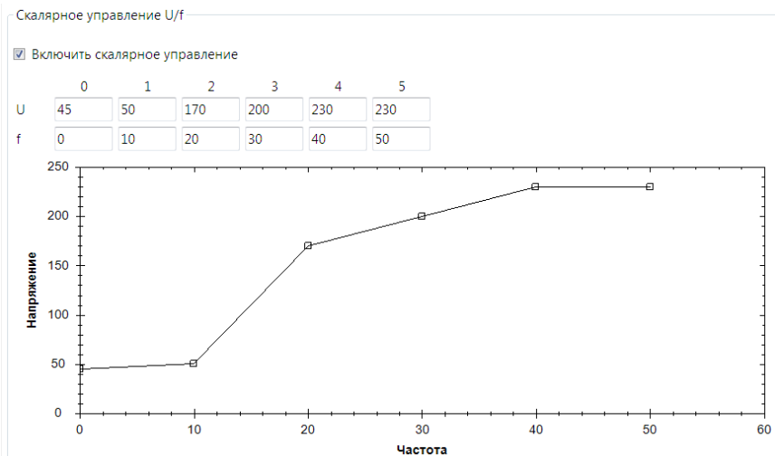
Рисунок 6.9 - Вид окна «Скалярное управление»
