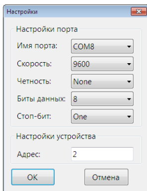
Рисунок 6.3 - Настройки связи ПЧВЗ И ПК
