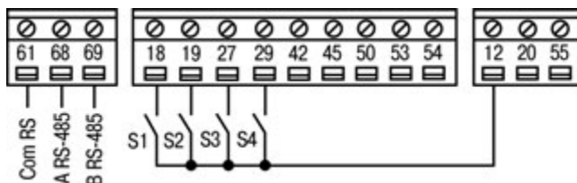
Рисунок 4.4 - Схема внешних подключений ПЧВЗ
