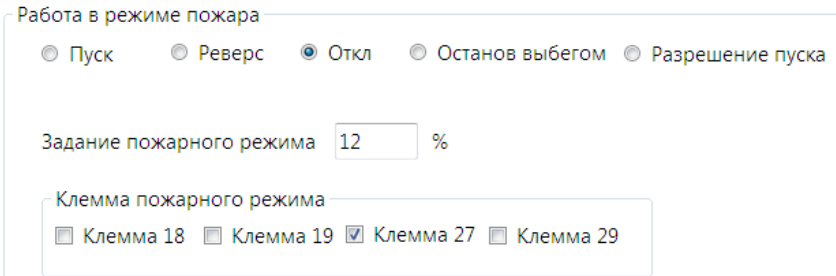
Рисунок 6.12 - Окно настройки «Пожарного режима»
