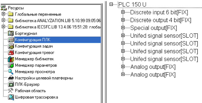
Рисунок 5.1 - Конфигурация ПЛК
