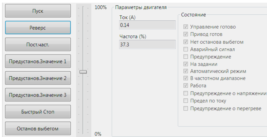
Рисунок 6.6 - Рабочее поле окна удаленного управления
