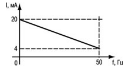
Рисунок 4.2 - Регулировочная характеристика ПЧВЗ
