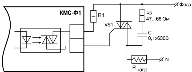
Рисунок 5.9 – Использование симисторной оптопары для управления силовым симистором
