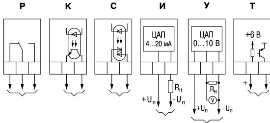
Рисунок 5.6 – Схемы подключения различных ВУ
