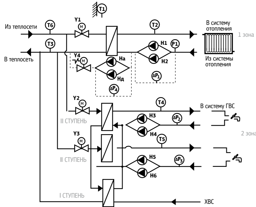
Типовая схема ИТП с двумя контурами ГВС и одним контуром отопления (по независимой схеме)
