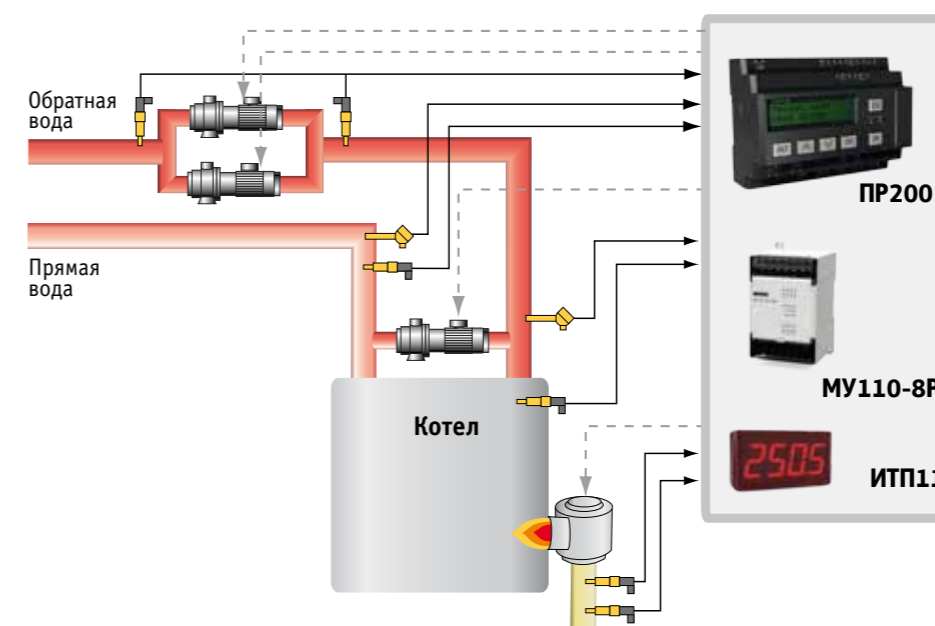
Пример спецификации оборудования ОВЕН для реализации функций
