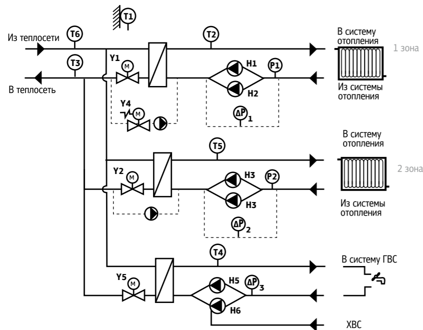
Типовая схема ИТП с двумя контурами отопления (по независимой схеме) и одним контуром ГВС
