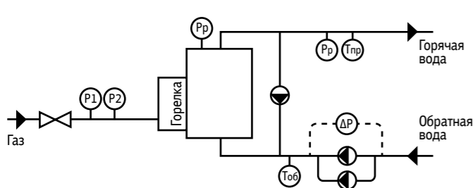
Типовая схема управления водогрейного котла
