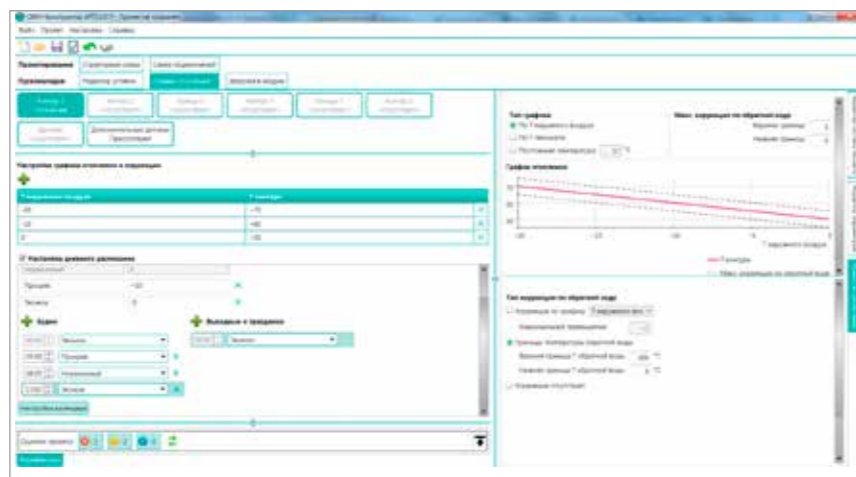
Окно конфигуратора на ПК после конфигурации
