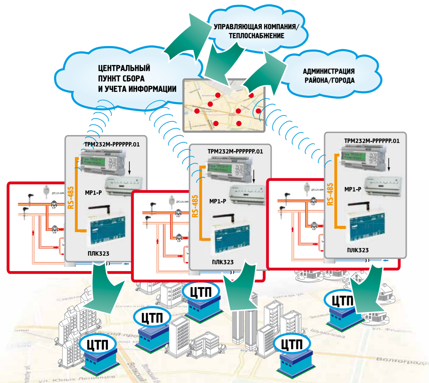
ПРИМЕР 12. Пример спецификации оборудования для комплексной автоматизации и диспетчеризации ИТП/ЦТП
