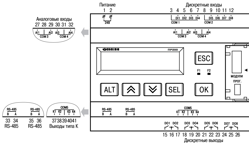
Рисунок А.15 – Расположение контактов ПР200-24.5.2.Х
