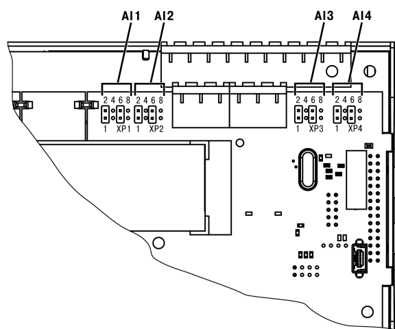
Рисунок 6.3 – Схема расположения переключек
