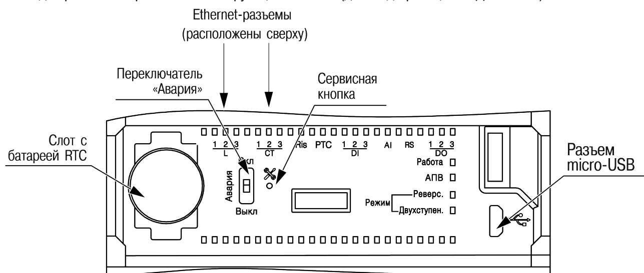
Рисунок 6.3 – Элементы под крышкой
