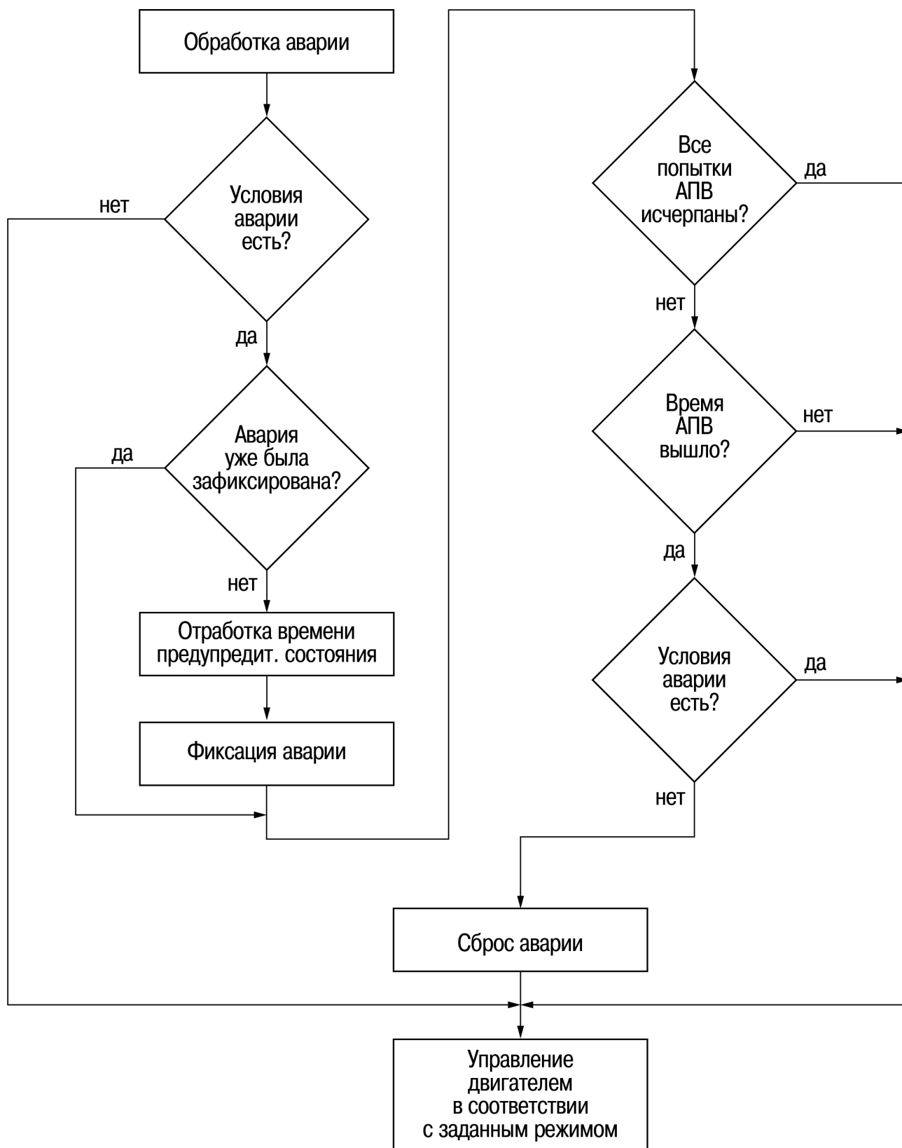
Рисунок 7.10 – Алгоритм обработки аварий с АПУ
