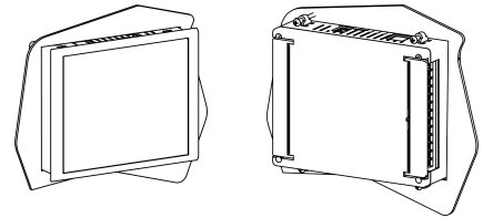
Рисунок 4.1 – Монтаж прибора щитового крепления
