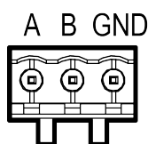
Рисунок 5.5 – Назначение контактов разъема RS-485-3
