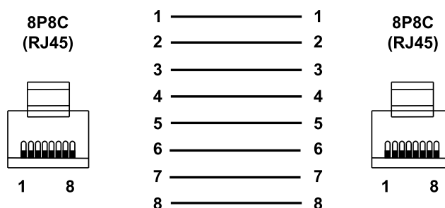
Рисунок 5.7 – Схема прямого кабеля для соединения прибора по сети Ethernet
