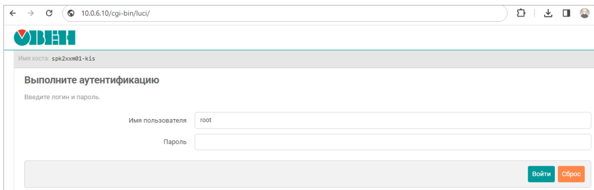
Рисунок 6.1 – Окно аутентификации
