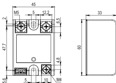
Рисунок 3 - габаритные и установочные размеры TTP серии RPS12
