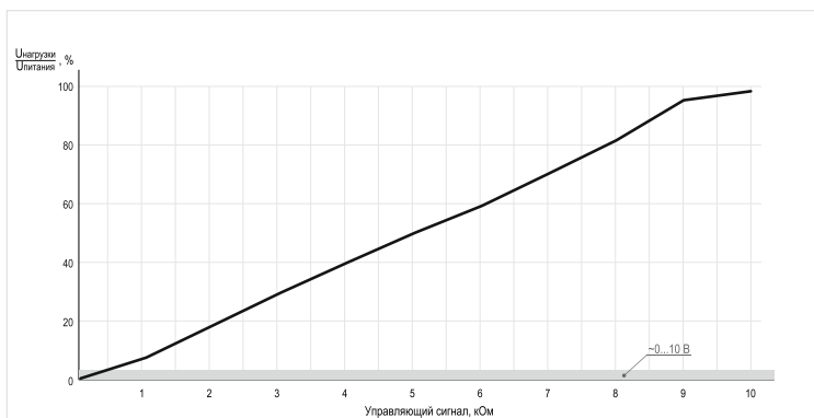
Рисунок 12 - выходная характеристика регуляторов RPS12-xx44 при управлении потенциометром 10 кОм
