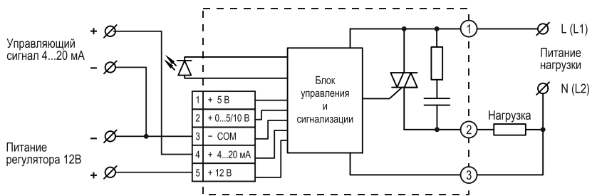
Рисунок 6 - схема подключения ТТР серии RPS12 при управлении сигналом тока 4...20 мА
