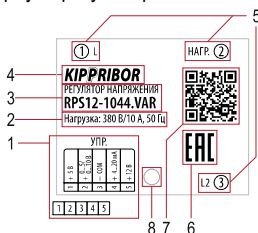
Рисунок 2 – заводская маркировка ТТР серии RPS12
