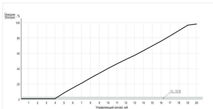
Рисунок 9 - выходная характеристика регуляторов RPS12-xx44 при управлении сигналом 0...20 мА
