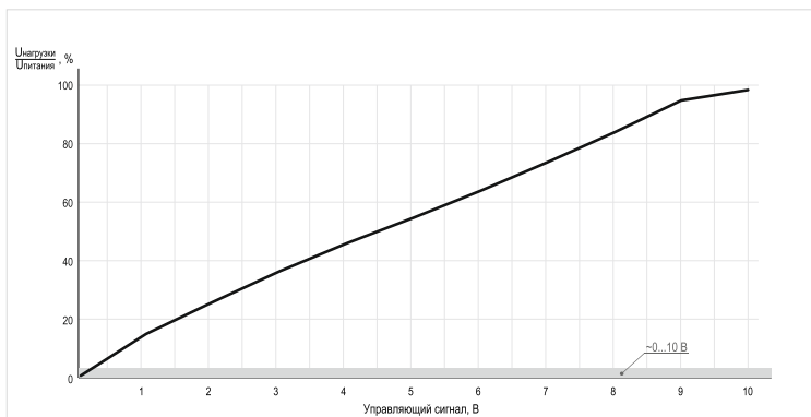
Рисунок 10 - выходная характеристика регуляторов RPS12-xx44 при управлении сигналом 0...10 В
