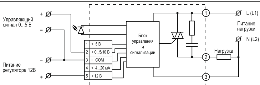
Рисунок 4 - схема подключения TTP серии RPS12 при управлении сигналом напряжения 0...5 В
