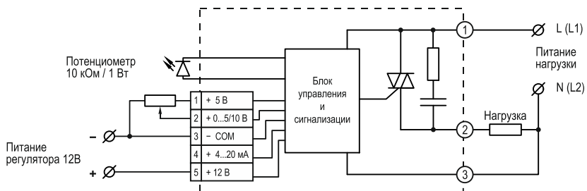
Рисунок 7 - схема подключения ТТР серии RPS12 при управлении потенциометром
