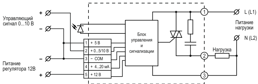
Рисунок 5 - схема подключения TTP серии RPS12 при управлении сигналом напряжения 0...10 В
