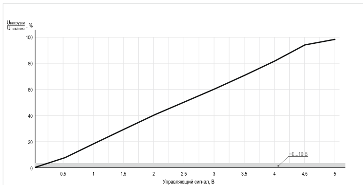
Рисунок 11 - выходная характеристика регуляторов RPS12-xx44 при управлении сигналом 0...5 В
