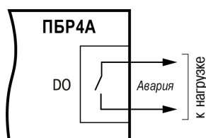
Рисунок 5.8 – Схема подключения дискретного выхода
