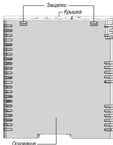
Рисунок 6.4 – Защелки крышки корпуса прибора
