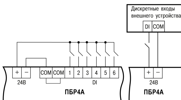
Рисунок 5.7 – Схема подключения дискретных входов с питанием от встроенного источника питания
