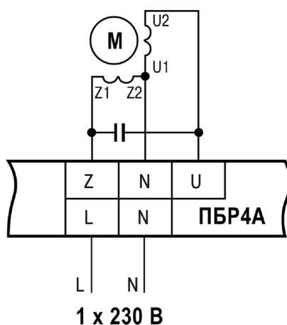
Рисунок 5.5 – Схемы подключения однофазного двигателя к ПБР4А-1
