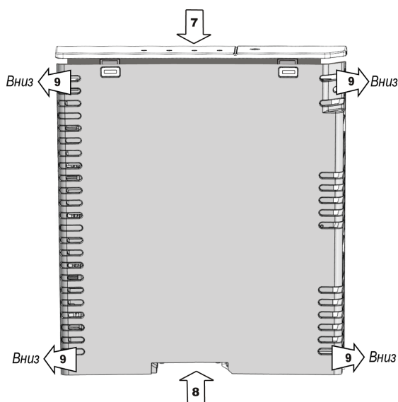
Рисунок 6.7 – Соединение крышки и основания корпуса
