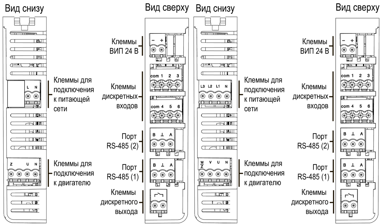
Рисунок 5.2 – Расположение клемм ПБР4А-1
