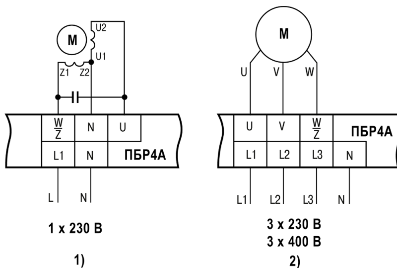
Рисунок 5.4 – Схемы подключения однофазного (1) и трехфазного (2) двигателей к ПБР4А-3
