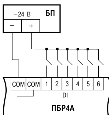
Рисунок 5.6 – Схема подключения дискретных входов с питанием от внешнего источника питания
