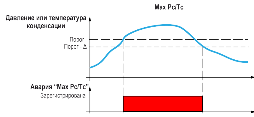
Рисунок 8.10 – Поясняющая диаграмма регистрации прибором аварии по превышению максимального порога давления или температуры конденсации
