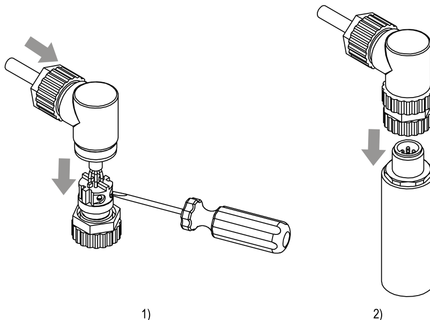
Рисунок 4.5 – Подключение датчика
