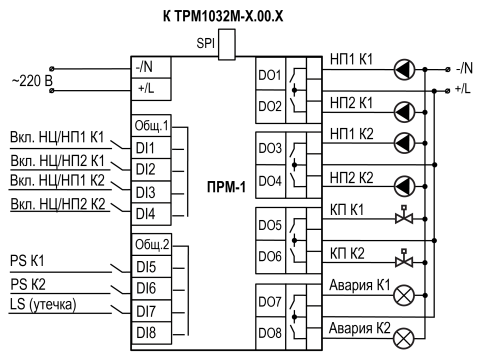
Рисунок 2 – Схема подключения контроллера
