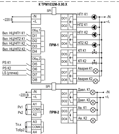
Рисунок 3 – Схемы подключения модулей расширения
