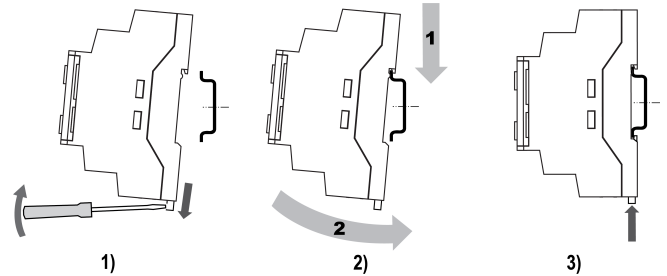
Рисунок 1 – Монтаж и демонтаж прибора
