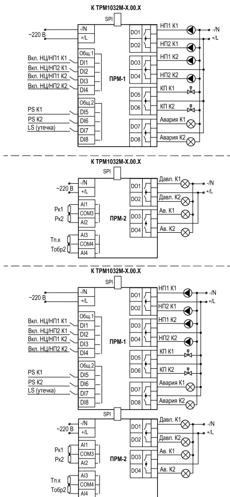
Рисунок 3 – Схемы подключения модулей расширения
