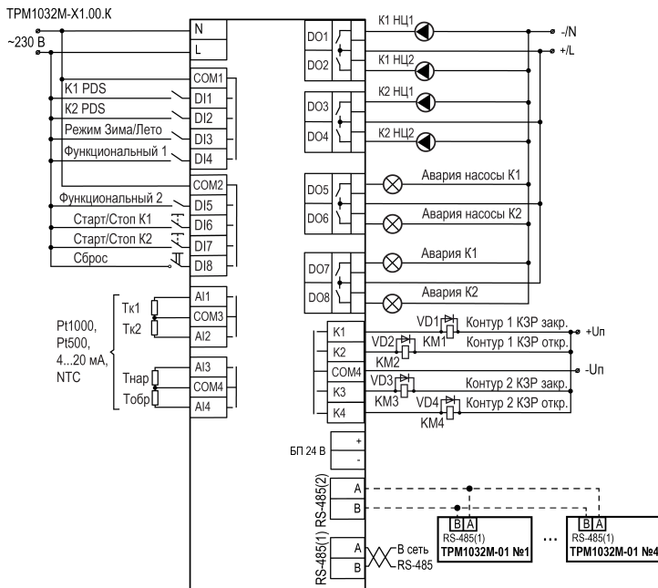
Рисунок 2 – Схема подключения контроллера
