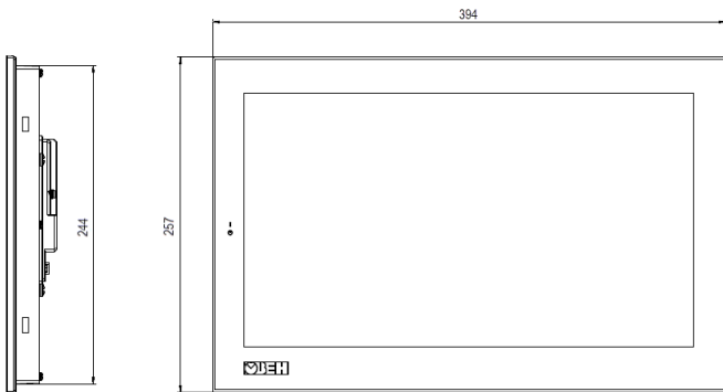
Рисунок 1 – Габаритные размеры СП210-15-Р
