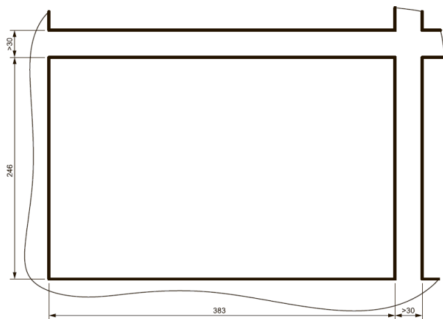
Рисунок 2 – Установочные размеры СП210-15-Р
