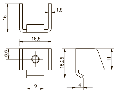
Рисунок 3 – Размеры крепежа
