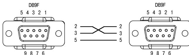
Рисунок 4 – Схема нуль-модемного кабеля для подключения по порту RS-232
