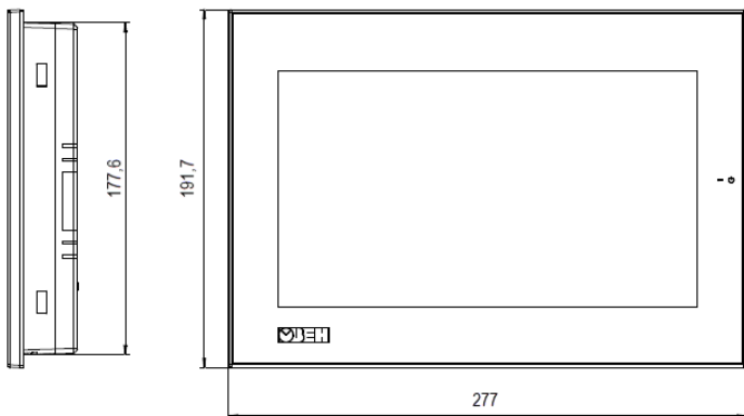
Рисунок 1 – Габаритные размеры СП210-10-Р
