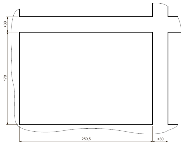
Рисунок 2 – Установочные размеры СП210-10-Р
