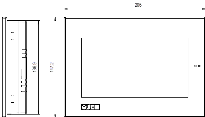
Рисунок 1 – Габаритные размеры СП210-07-Р
