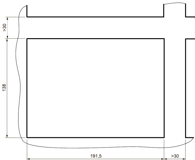
Рисунок 2 – Установочные размеры СП210-07-Р
