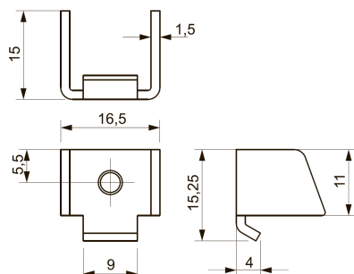
Рисунок 3 – Размеры крепежа
