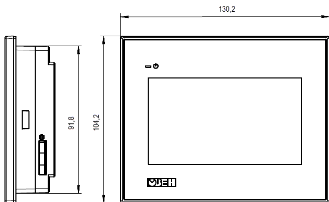
Рисунок 1 – Габаритные размеры СП210-05-Р
