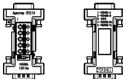
Рисунок 5 – Внешний вид адаптера СП210
