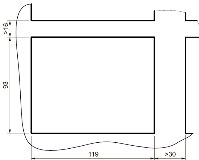
Рисунок 2 – Установочные размеры СП210-05-Р
