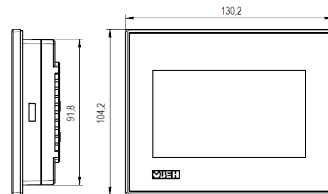
Рисунок 1 – Габаритные размеры СП210-05-Б
