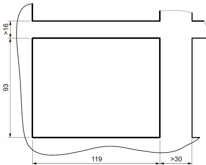
Рисунок 2 – Установочные размеры СП210-05-Б
