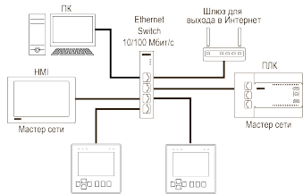
Рисунок 11 – Подключение по схеме «Звезда»
