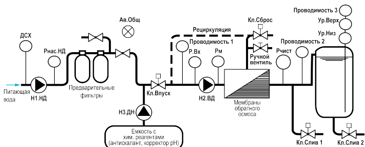
Рисунок 1 – Объект управления
