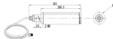
Рисунок 3 – Габаритные размеры датчика в автоматическом очистном устройстве
