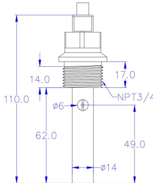
Рисунок 4 – Проточный электрод из нержавеющей стали (резьба G3/4)
