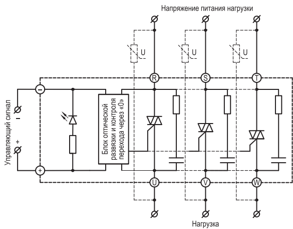
Схема включения ТТР серии HT-xx44.ZD3 (выходы - симисторы (TRIAK))
