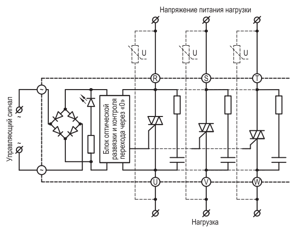
Схема включения ТТР серии HT-xx44.ZA2 (выходы – симисторы (TRIAK))
