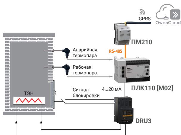
Пример применения регулятора мощности при управлении температурой печи нагрева
