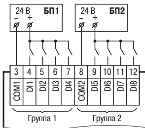
Подключение дискретных датчиков =24 В с выходом типа «сухой контакт» (для модификаций ПР200-24, ПР200-220.2x)
