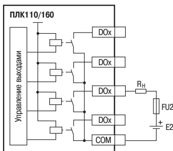
Подключение цепей защиты при активной нагрузке, RH – пользовательская нагрузка (двигатель, нагреватель, контактор и т.д.)
