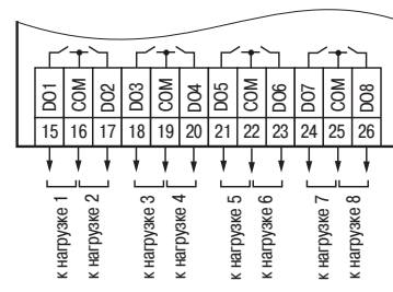
Подключение дискретных выходов типа Р
