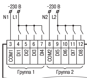
Подключение дискретных датчиков ~230 В с выходом типа «сухой контакт» (для модификаций ПР200-220, кроме ПР200-220.2x)
