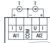
Подключение датчиков с токовым выходом
