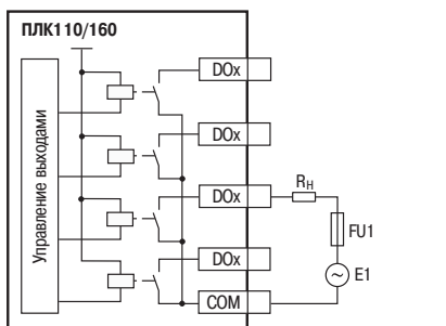
Подключение цепей защиты при активной нагрузке, RH – пользовательская нагрузка (двигатель, нагреватель, контактор и т.д.)
