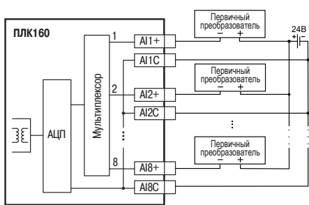
Схема подключения к аналоговым входам ПЛК160 унифицированных сигналов тока/напряжения
