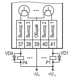
Подключение дискретных выходов типа К ПР200-х.5, ПР200-220.25
