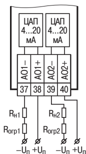
Подключение аналоговых выходов типа И ПР200-х.2, ПР200-220.22
