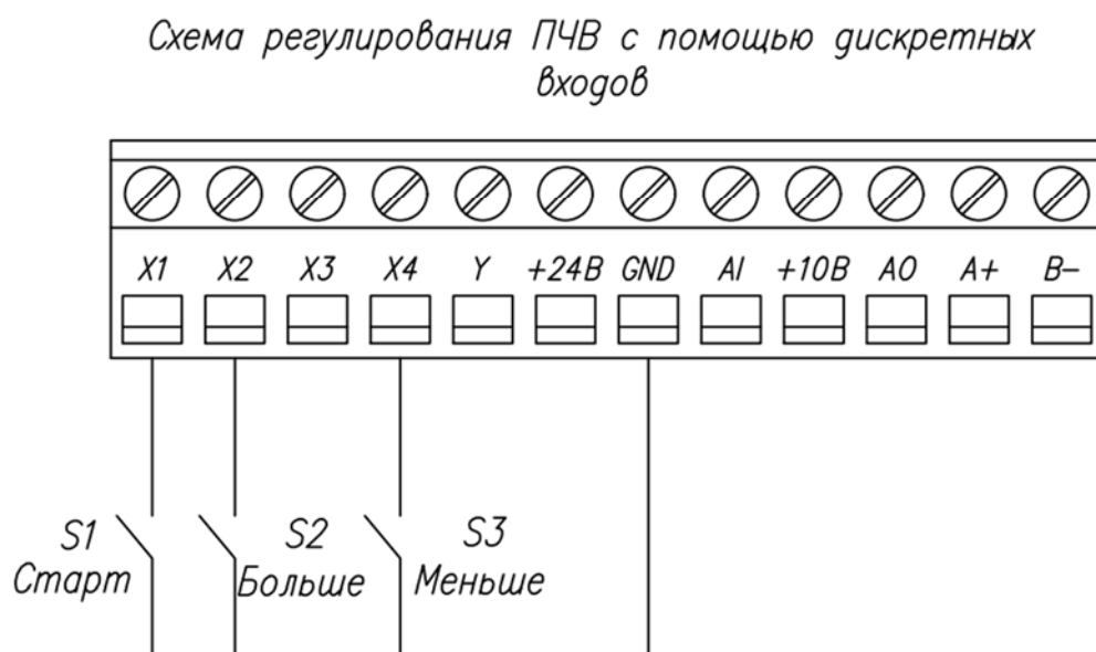
Рисунок 1. Схема подключения для работы в режиме управления по дискретным входам
